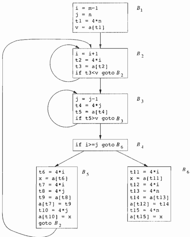
图 9-3 快速排序代码片断的流图
