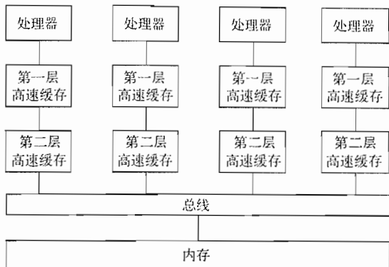
图 11-1 对称多处理器体系结构
