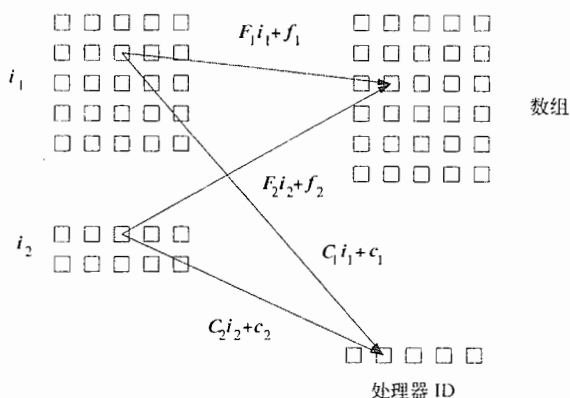
图 11-25 空间分划约束
