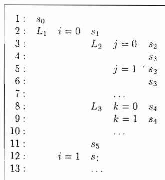
图 11-45 例 11.53 中的程序的执行顺序
