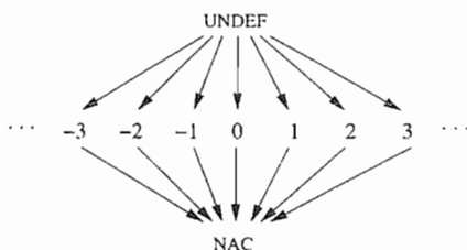
图 9-25 表示了一个整数类型变量的所有可能“取值”的半格
