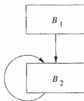
图 9-19 将 OUT 集合初始化为 \emptyset 局限性太大
