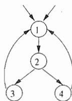
图 9-46 具有相同循环头的两个循环
