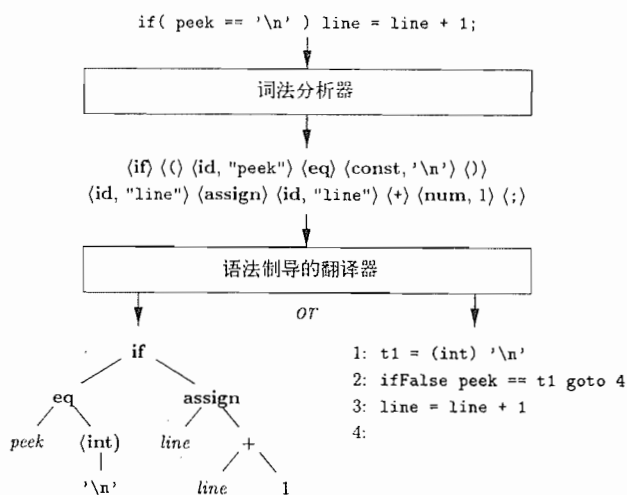
图 2-46 一个语句的两种可能的翻译结果
