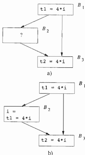
图 9-17 跨越多个基本块的潜在的公共子表达式
