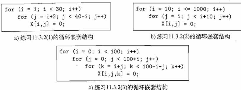
图 11-17 练习 11.3.2 的循环嵌套结构
