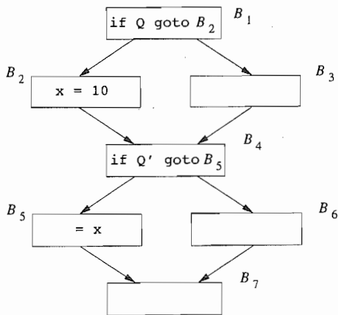
图 9-29 UNDEF 和一个常量值的交汇运算值
