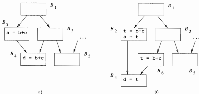
图 9-31 B_3 \rightarrow B_4 是一条关键边
