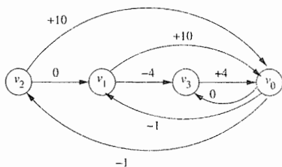
图 11-21 例子 11.37 中的约束的图形表示
