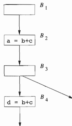
图 9-35 例 9.31 的流图,用以说明可用表达式的使用
