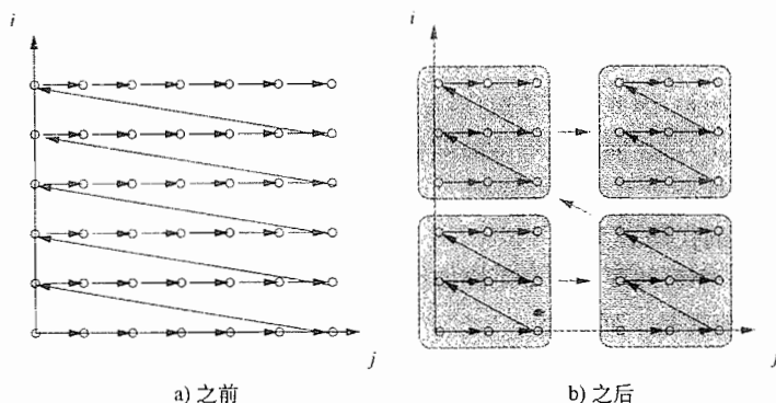
图 11-56 在一个深度为 2 的循环嵌套结构分块之前和分块之后的执行顺序
