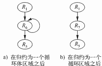
图 9-49 把图 9-48 的流图归约为单个区域的步骤
