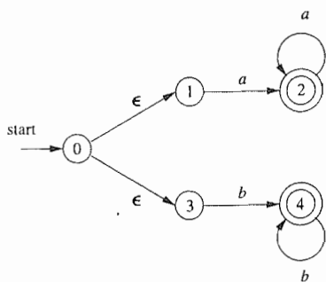
图 3-26 接受 aa^*|bb^* 的 NFA
