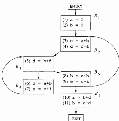
图 9-10 练习 9.1.1 的流图
