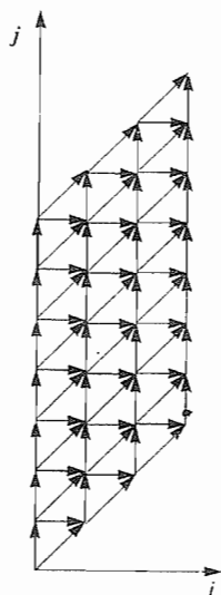
d) 图 11-51c 中代码的数据依赖关系
