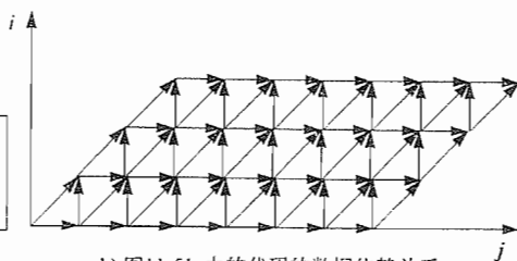
b) 图 11-51a 中的代码的数据依赖关系
