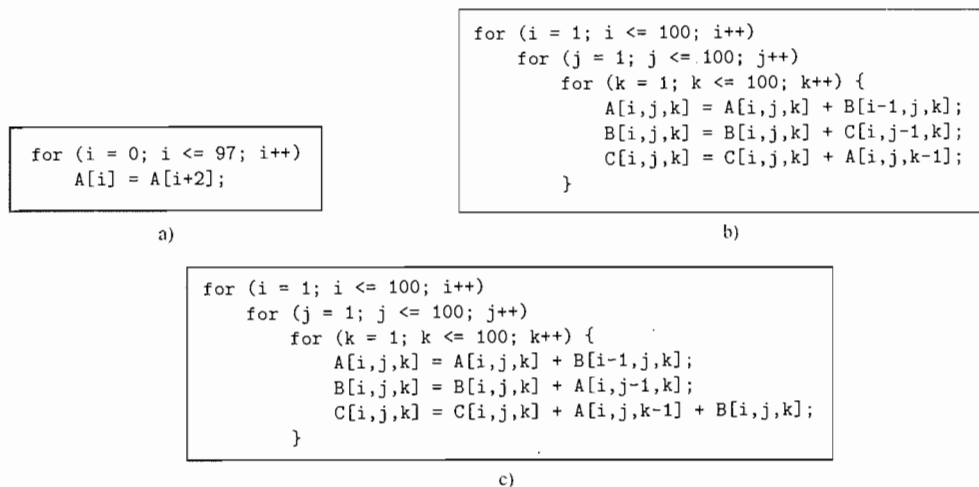
图 11-37 练习 11.7.2 的代码
