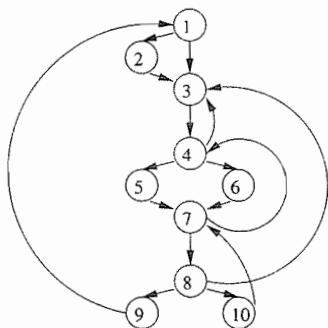
图 9-38 一个流图
