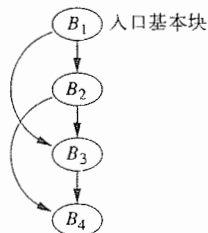
图 9-47 区域的例子
