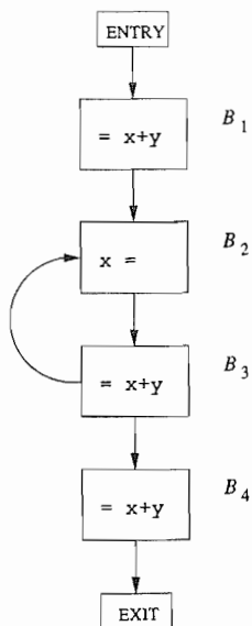
图 9-37 练习 9.5.1 的流图
