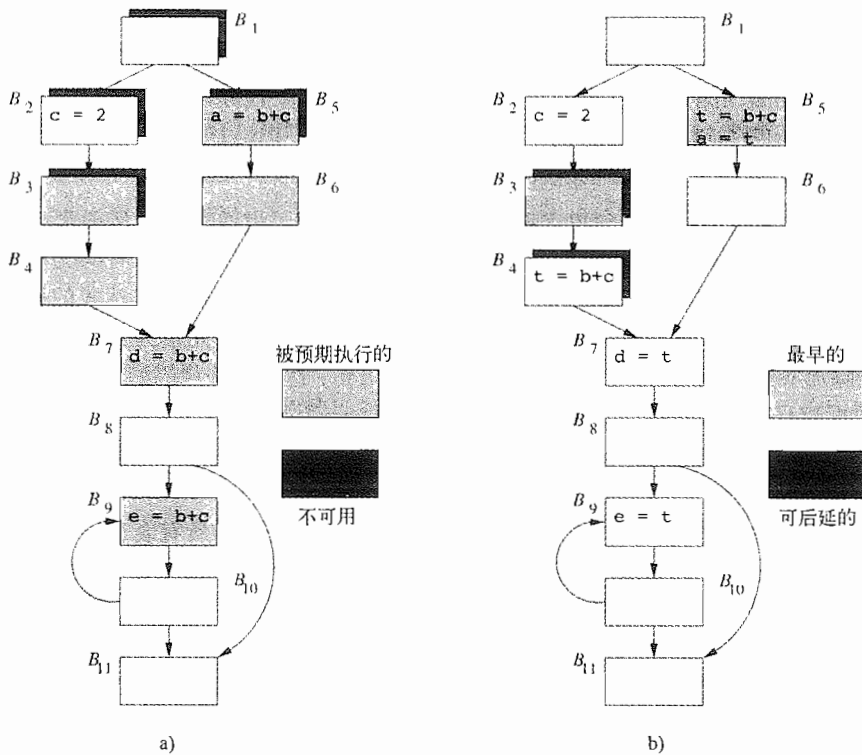
图 9-33 例 9.30 的流图
