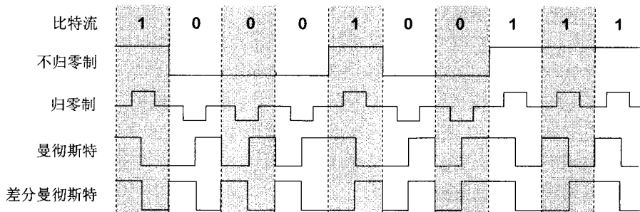
图 2-2 数字信号常用的编码方式
