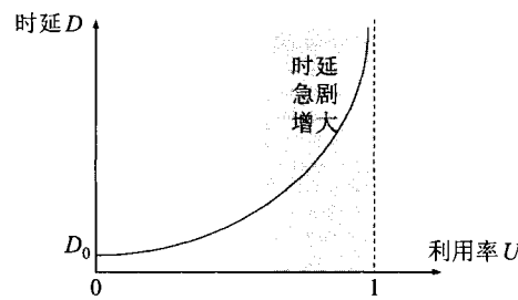
图 1-16 时延与利用率的关系
