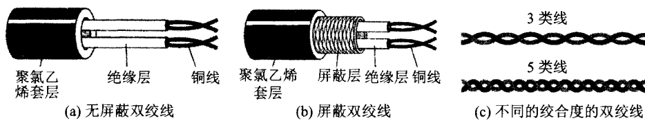
图 2-6 双绞线的示意图
