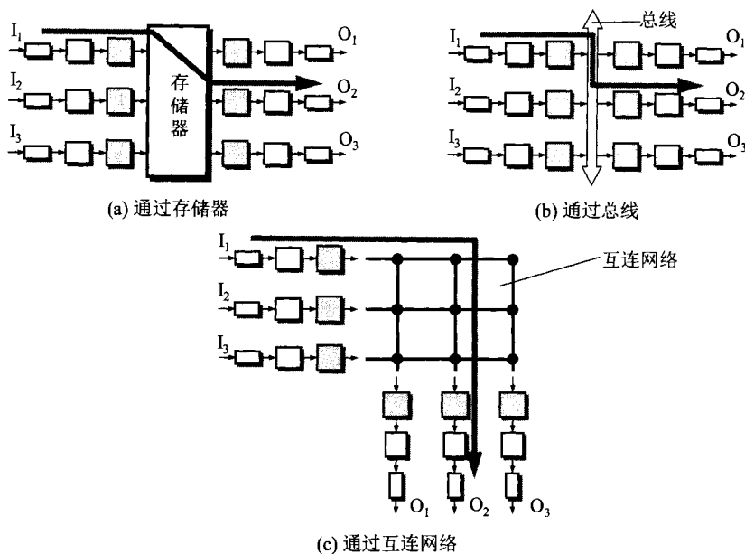
图 4-45 三种常用的交换方法
