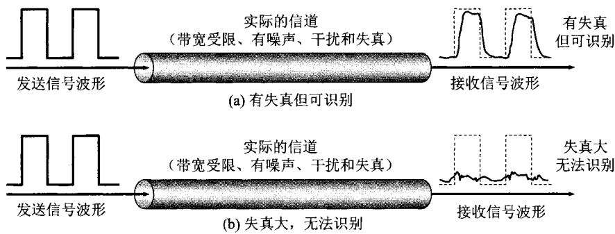
图 2-4 数字信号通过实际的信道
