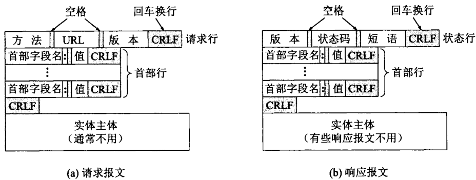
图 6-12 HTTP 的报文结构
