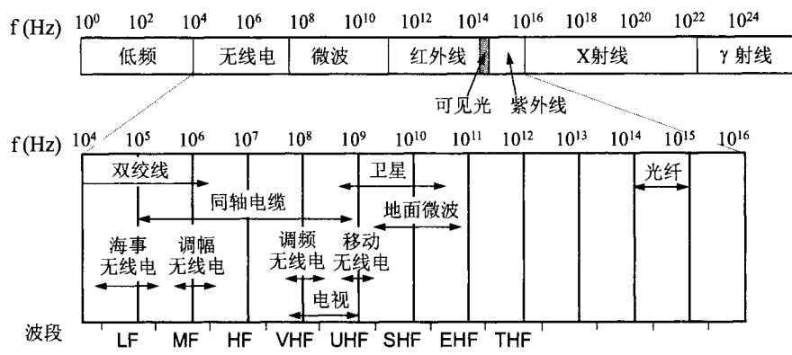
图 2-5 电信领域使用的电磁波的频谱
