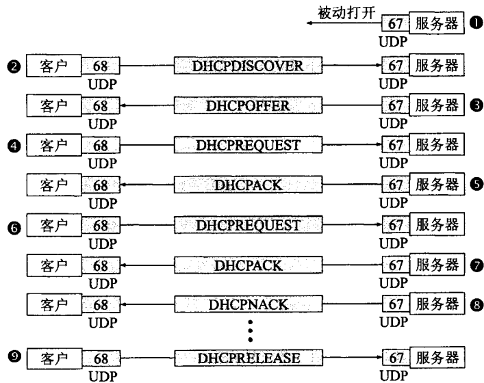
图 6-20 DHCP 协议的工作过程
