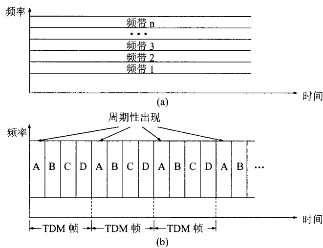
图 2-14 频分复用(a)和时分复用(b)
