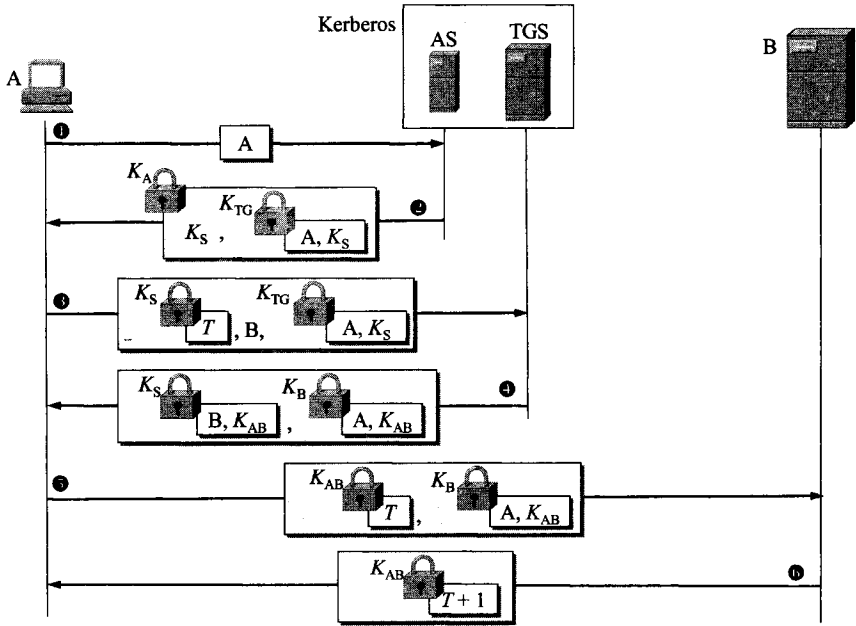
图 7-12 Kerberos 的工作原理
