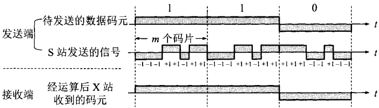
图 2-18 CDMA 的工作原理
