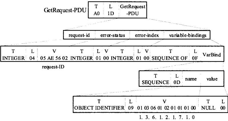
图 6-26 GetRequest-PDU 的 ASN.1 编码
