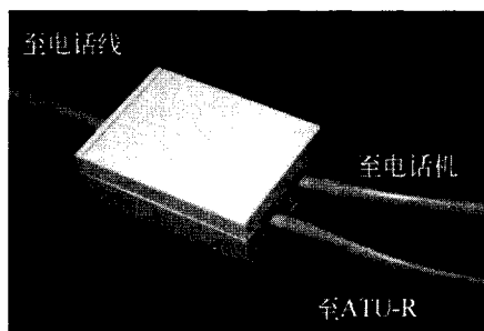
图 2-22 电话分离器（有三个 RJ-11 插口）
