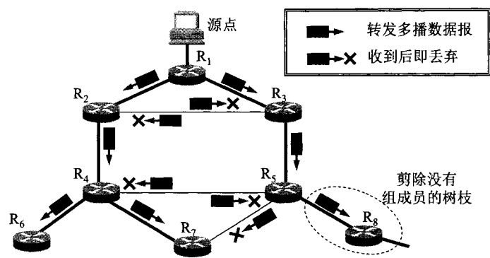
图 4-57 反向路径广播 RPB 和剪除
