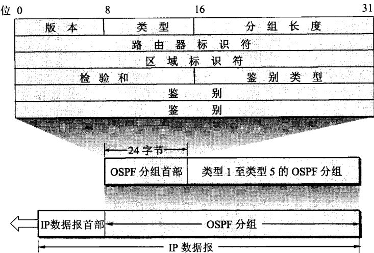
图 4-35 OSPF 分组用 IP 数据报传送
