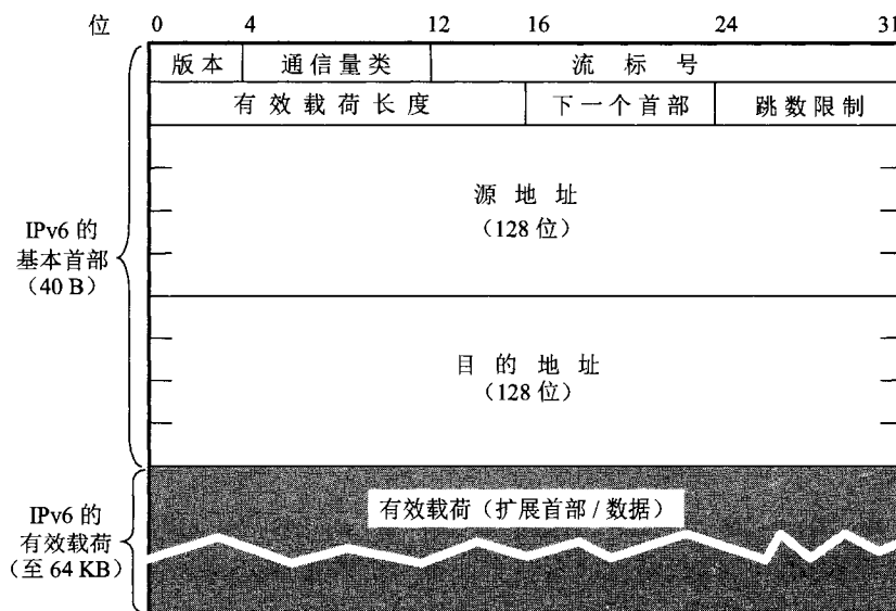
图 4-47 40 字节长的 IPv6 基本首部
