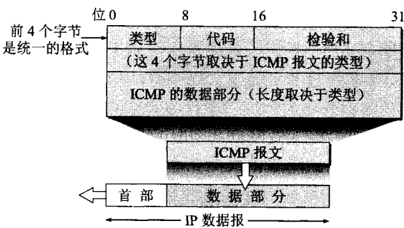
图 4-27 ICMP 报文的格式
