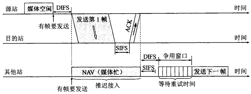
图 9-6 CSMA/CA 协议的工作原理
