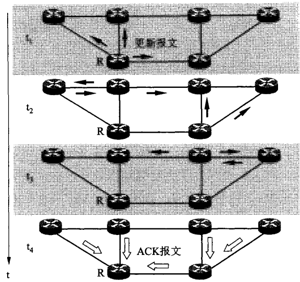
图 4-37 用可靠的洪泛法发送更新分组
