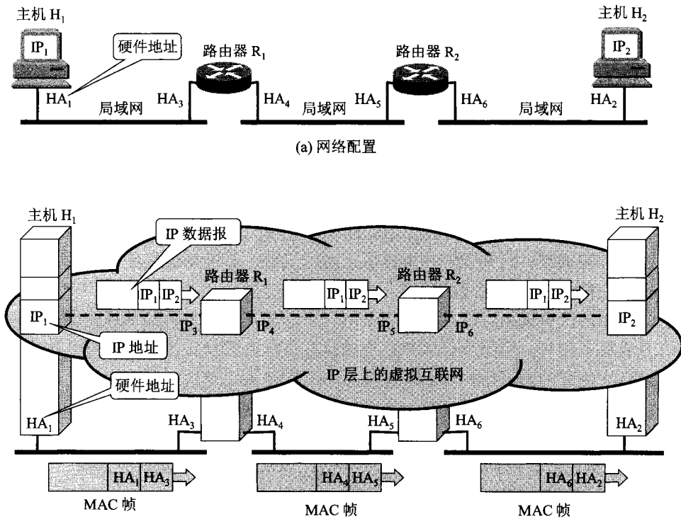
(b) 不同层次、不同区间的源地址和目的地址
