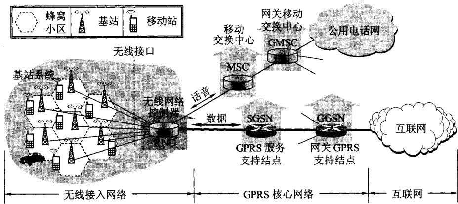
图 9-17 3G 蜂窝通信系统的重要组成构件
