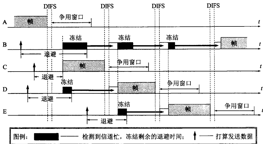
图 9-7 802.11 的退避机制的概念
