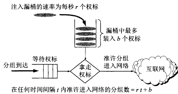
图 8-22 漏桶管制器的工作原理
