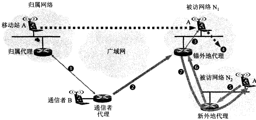
图 9-19 使用直接路由选择向移动站发送数据报
