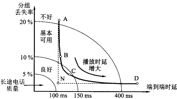
图 8-10 播放时延有一个最佳值
