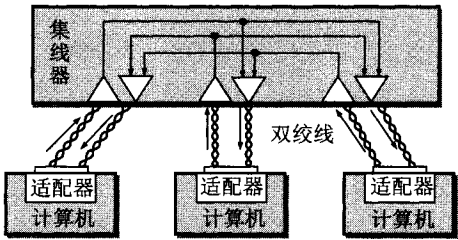
图 3-20 具有三个接口的集线器
