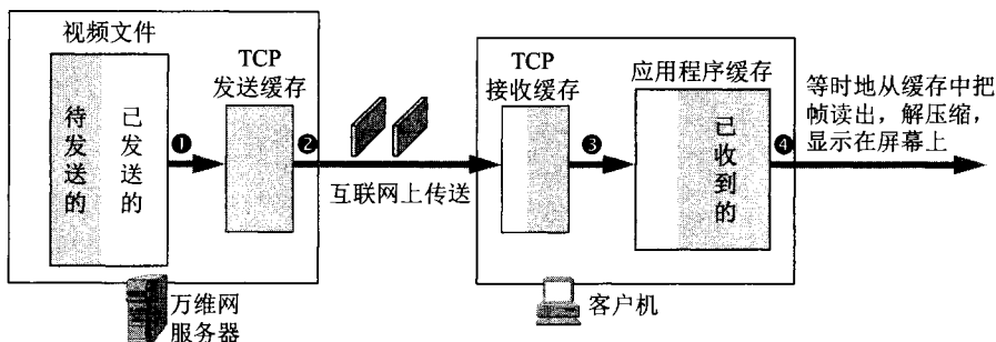
图 8-7 使用 TCP 传送流式视频的主要步骤
