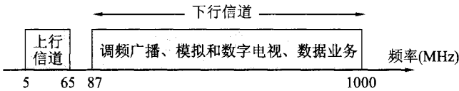
图 2-24 我国的 HFC 网的频带划分
