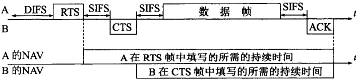
图 9-8 发送 RTS 帧和 CTS 帧对信道进行预约
