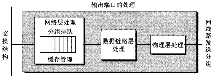
图 4-44 输出端口把交换结构传送过来的分组发送到线路上
