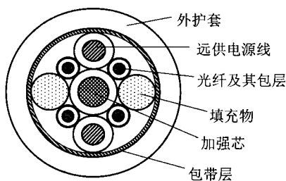
图 2-11 四芯光缆剖面的示意图
