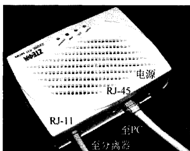
图 2-21 ADSL 调制解调器(ADSL ATU-R)
