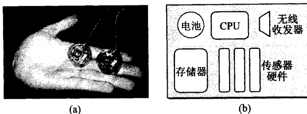
图 9-3 传感器结点的形状(a)和组成(b)
