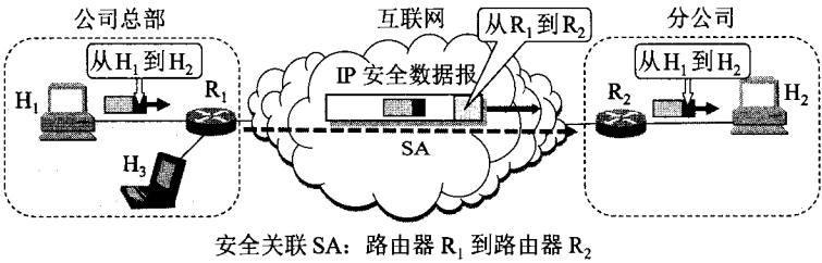
图 7-13 安全关联 SA 的示意图
