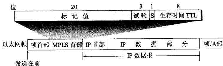
图 4-64 MPLS 首部的格式
