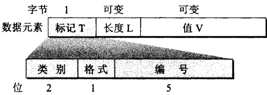
图 6-23 用 TLV 方法进行编码
