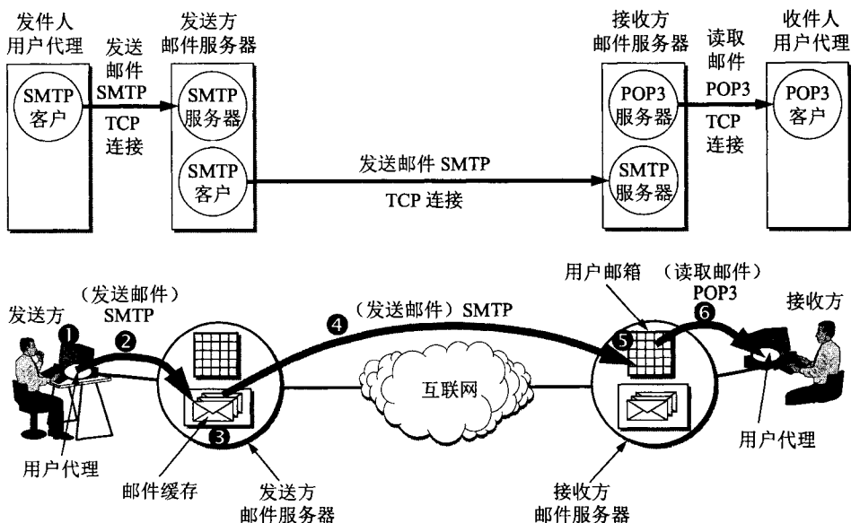
图 6-17 电子邮件的最主要的组成构件
