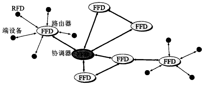
图 9-15 ZigBee 的组网方式
