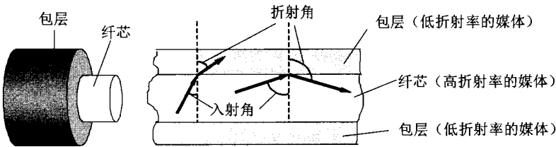
图 2-8 光线在光纤中的折射
