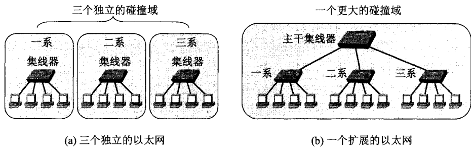
图 3-24 用多个集线器连成更大的以太网
