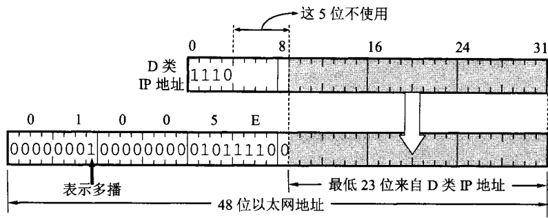
图 4-54 D 类 IP 地址与以太网多播地址的映射关系
