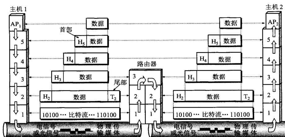
图 1-19 数据在各层之间的传递过程
