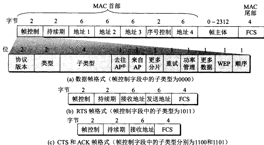
图 9-10 802.11 局域网的帧格式
