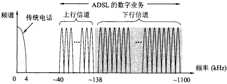
图 2-19 DMT 技术的频谱分布
