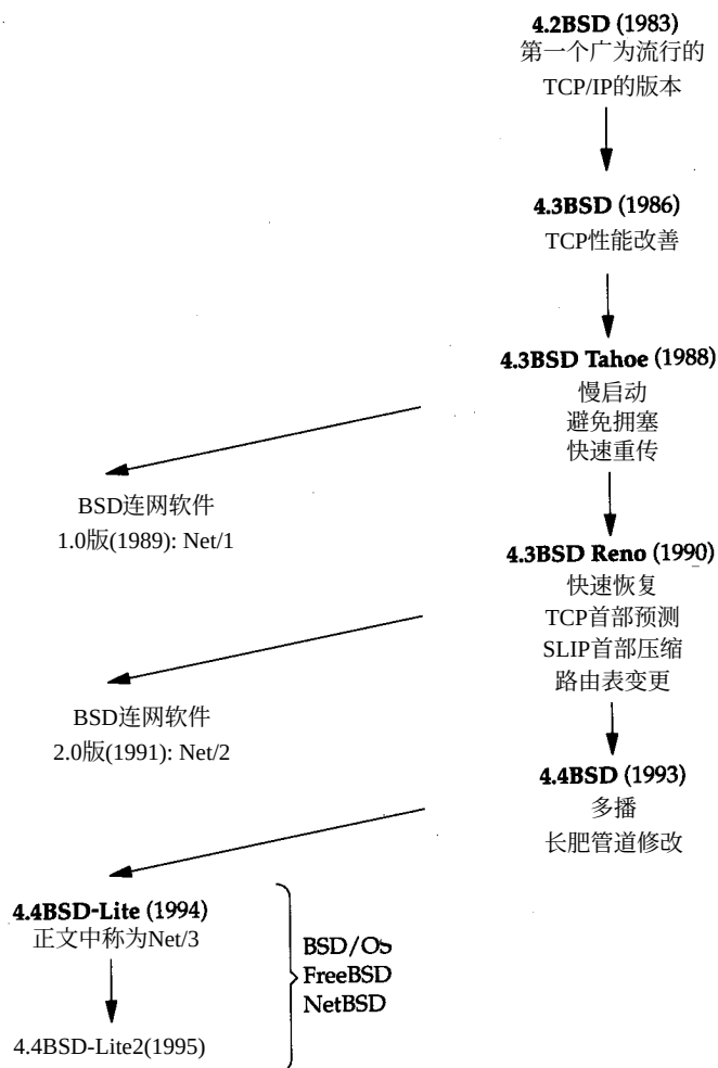
图1-16 带有重要TCP/IP特性的各种BSD发行
