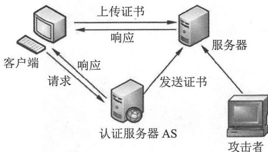
图5-55 Kerberos工作机制
