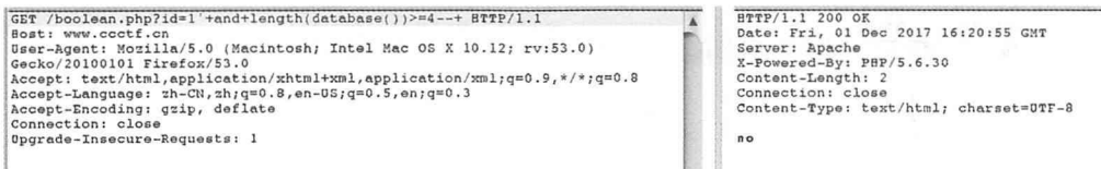
图4-24 判断数据库库名的长度（3）
