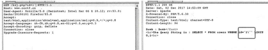
图4-46 单引号被转义
