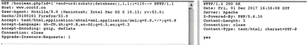
图4-27 利用ord判断数据库库名
