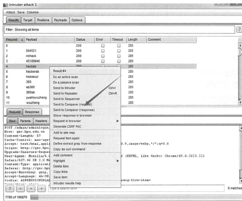
图3-43 数据加载
