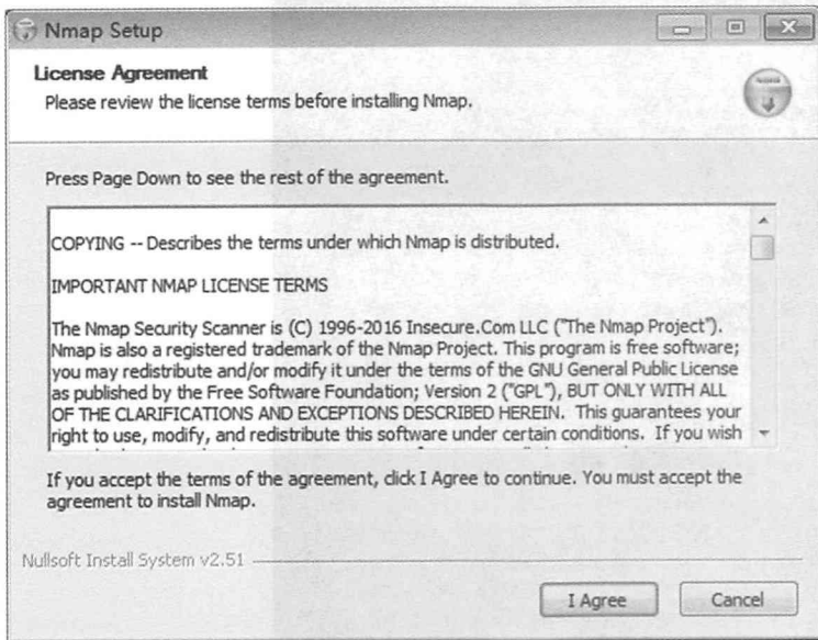
图3-46 安装Nmap
