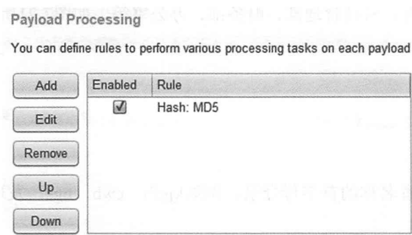
图7-23 MD5哈希
