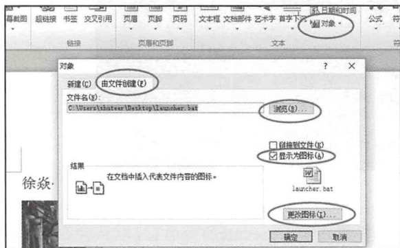
图6-82 插入新对象
