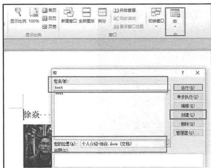
图6-88 创建宏
