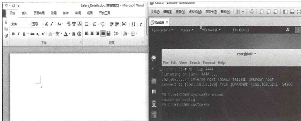
图6-197 反弹成功
