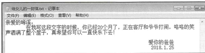
图6-112 输入文字
