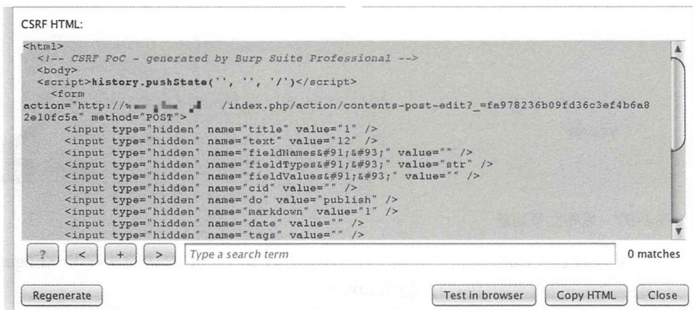
图4-99 Burp生成的HTML代码
