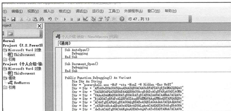
图6-89 复制宏代码
