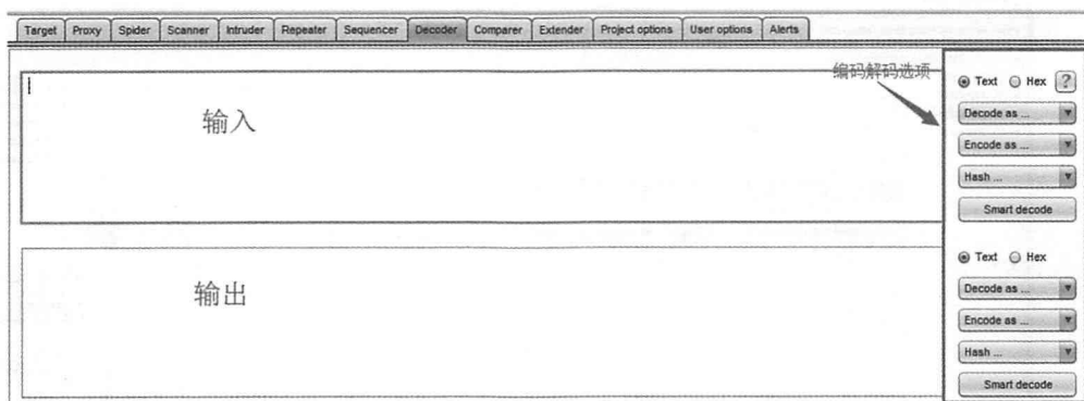
图3-25 Decoder的界面
