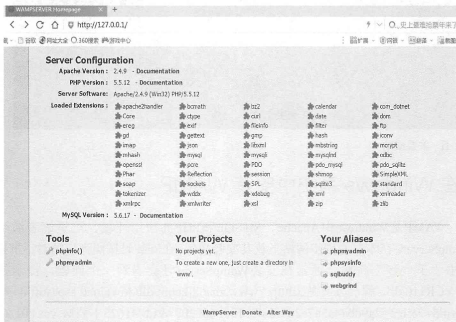
图2-8 访问127.0.0.1
