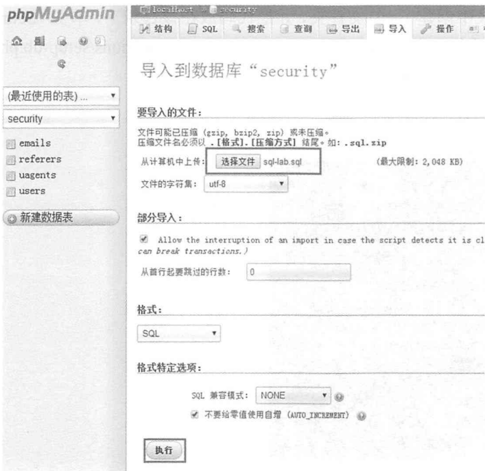
图2-13 导入数据库
