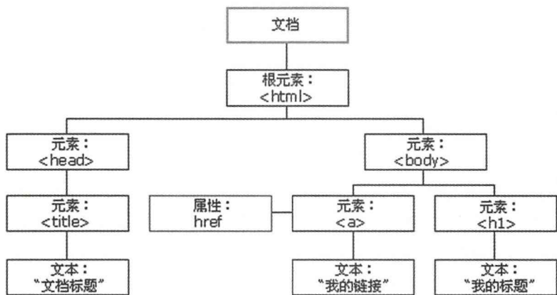
图4-80 HTML DOM树
