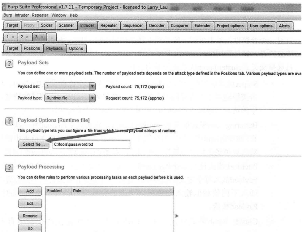
图3-37 选中字典
