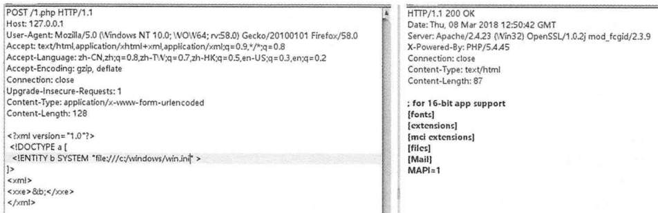
图4-124 读取文件
