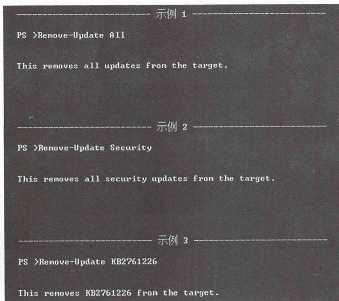
图6-185 示例说明
