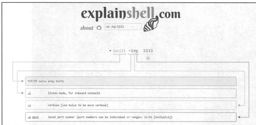
图6-177 网站截图
