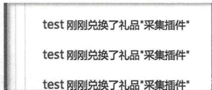
图7-18 成功执行（2）
