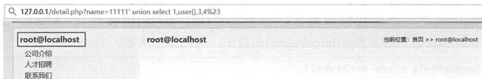
图7-2 注入成功
