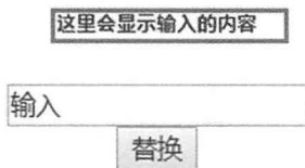
图4-88 HTML页面
