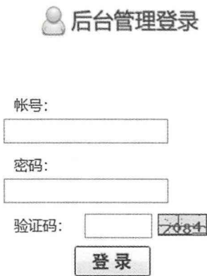
图7-19 登录界面
