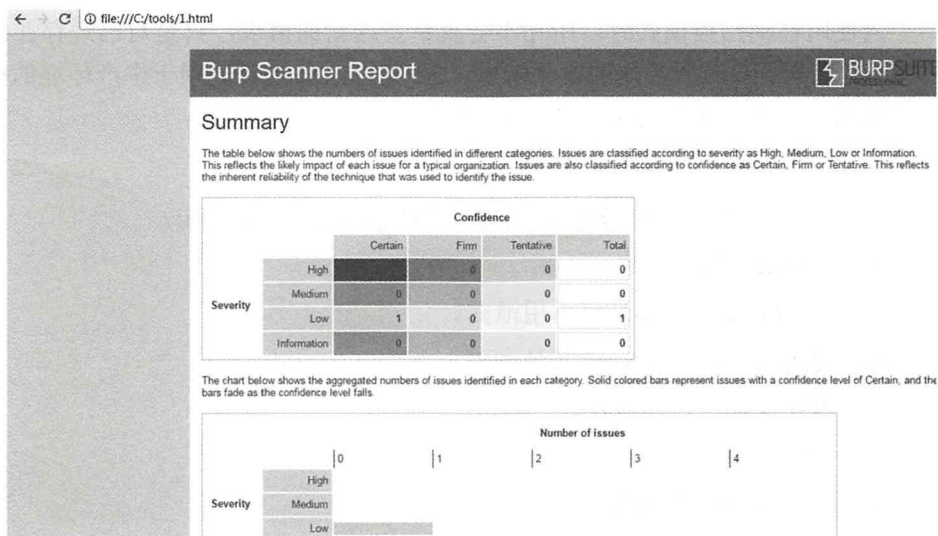
图3-31 扫描结果
