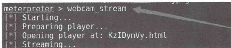
图5-35 抓取视频
