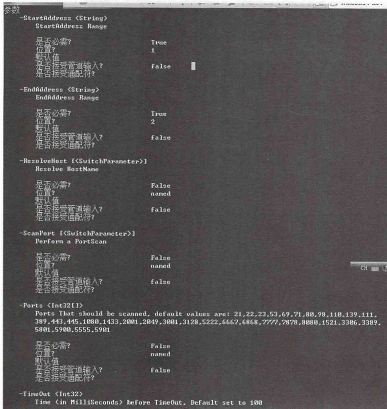
图6-188 查看帮助信息
