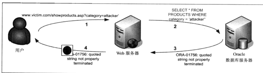
图 2-5 产生 SQL 注入错误的过程中的信息流
