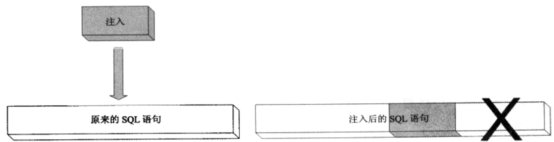
图 2-14 终止式 SQL 注入
