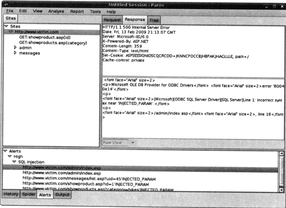
图 2-21 Paros Proxy
