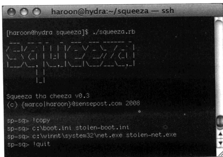
图 6-10 从远程服务器复制一个二进制文件
