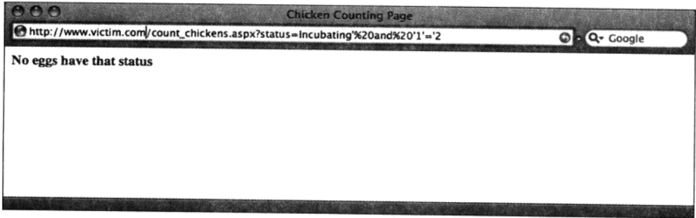
图 5-3 强制产生一个空结果集
