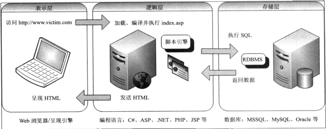
图 1-1 简单的三层架构
