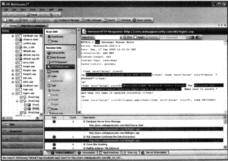
图 2-17 HP WebInspect
