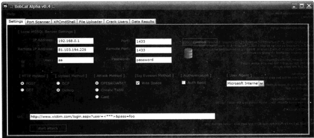
图 4-18 Bobcat 的截图
