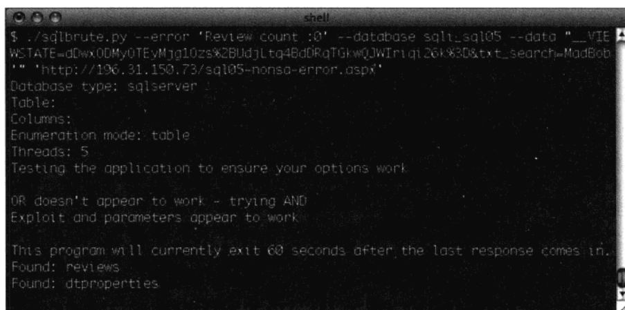
图 5-14 运行 SQLBrute
