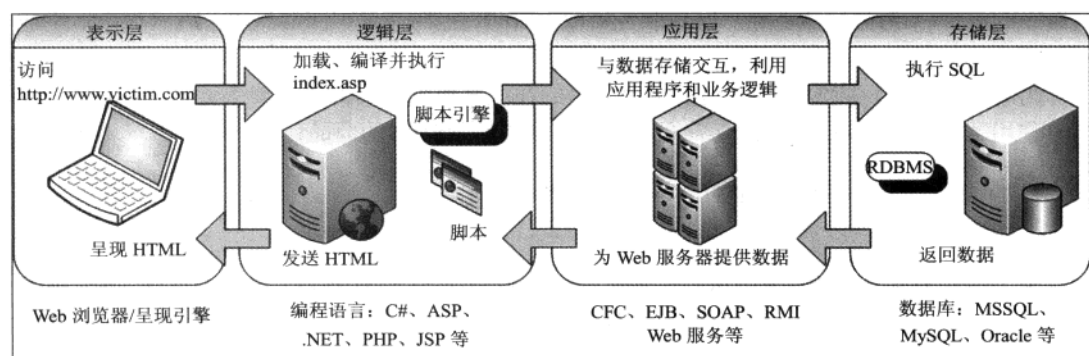
图 1-2 四层架构
