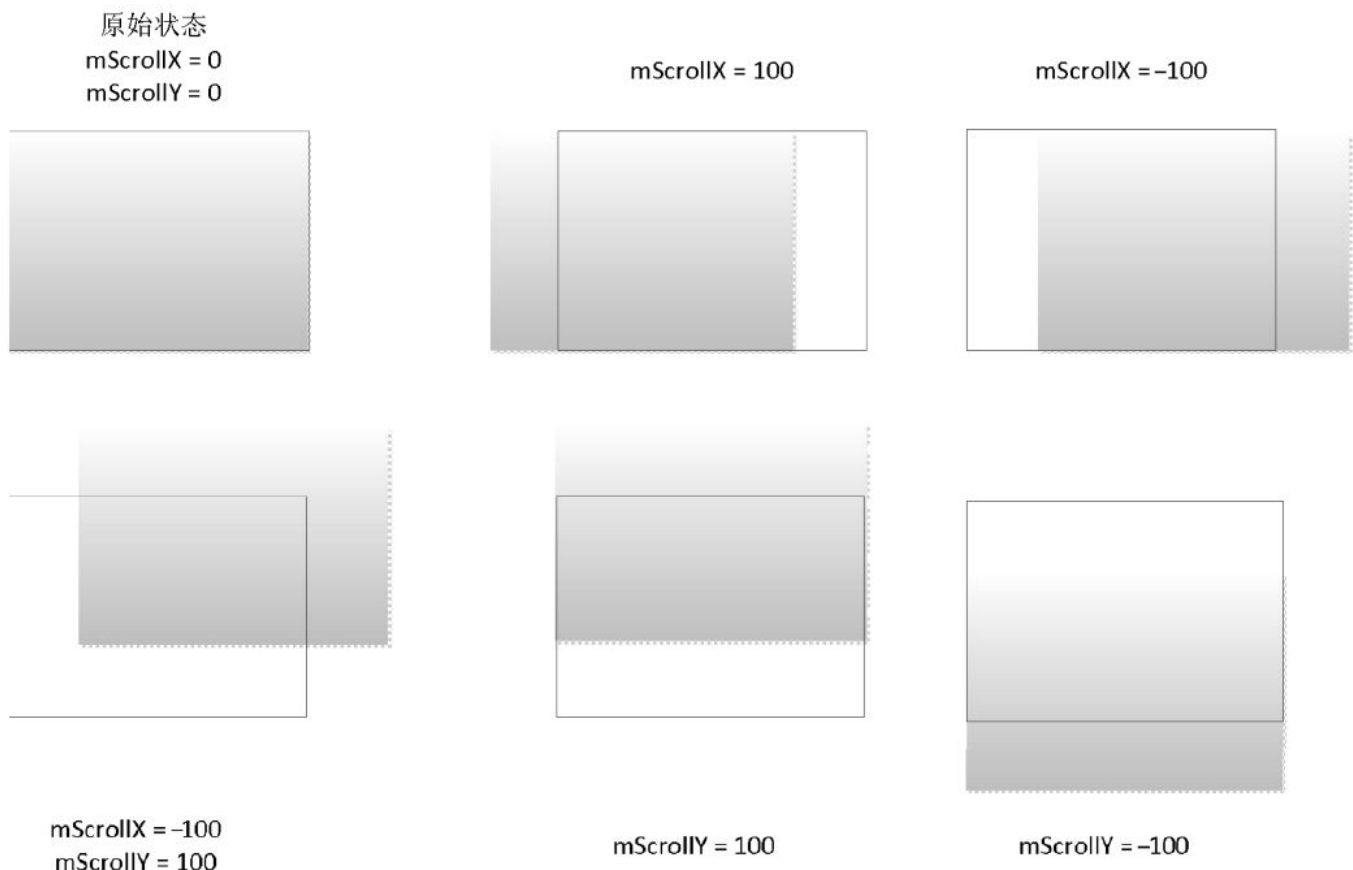
圖3-3 mScrollX 與 mScrollY 的取值範圍
