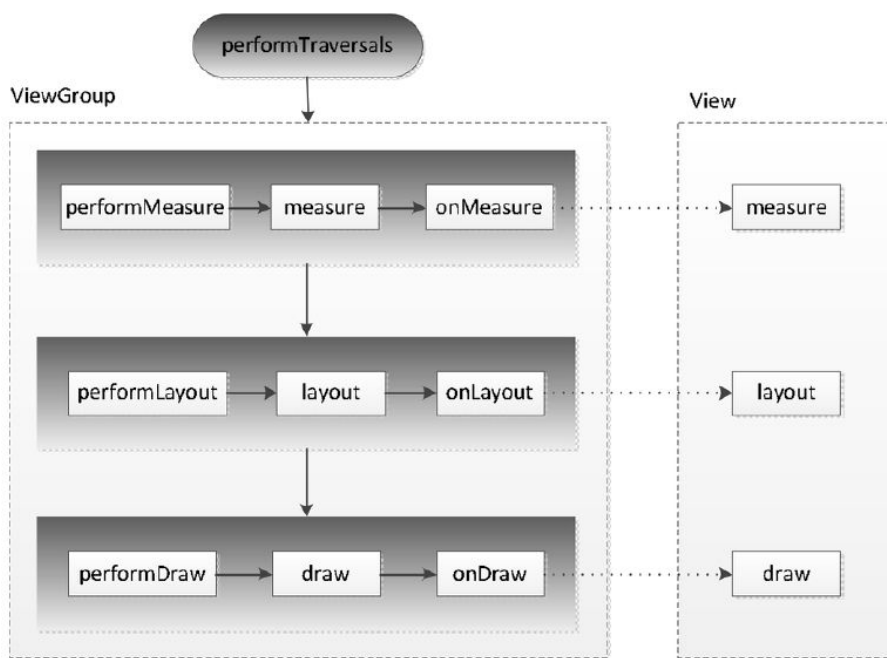
图4-1 performTraversals的绘制流程
