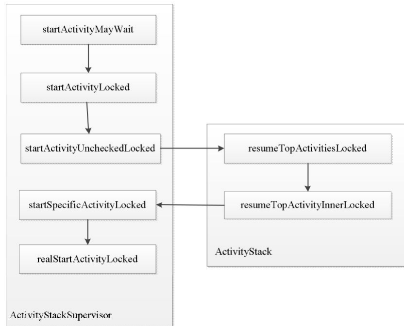
图9-1 Activity启动过程在ActivityStackSupervisor和ActivityStack之间的传递顺序
