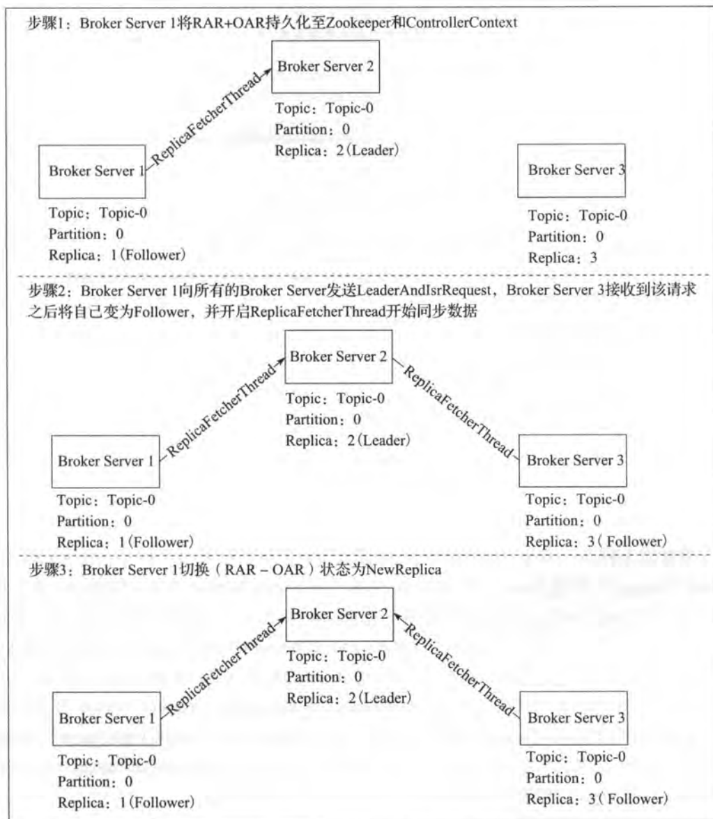
图 5-6 分区重分配阶段一
