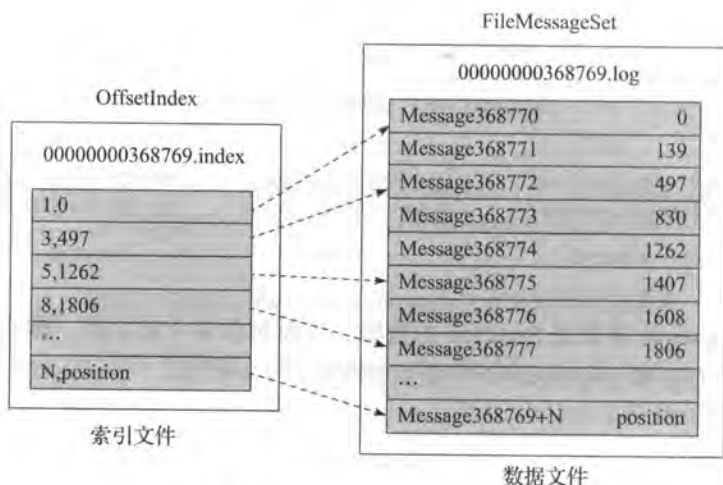
图 4-5 FileMessageSet 和 OffsetIndex 的关系
