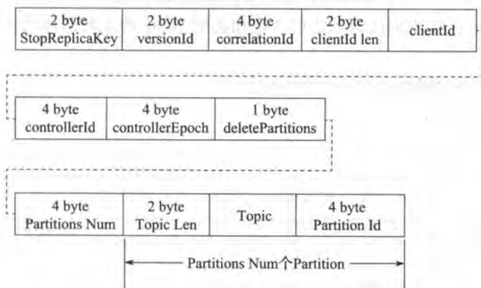
图 4-22 StopReplicaRequest 二进制数据组成
