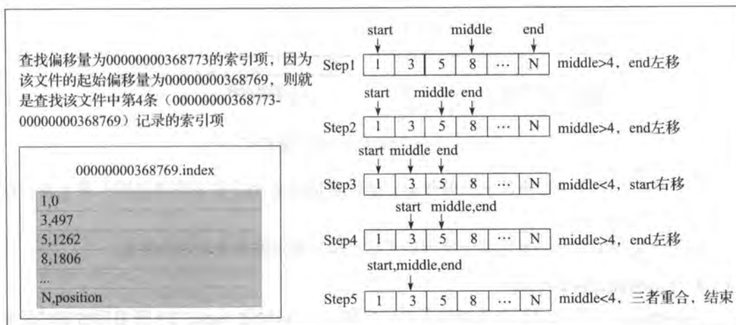
图 4-7 二分查找算法查找索引项
