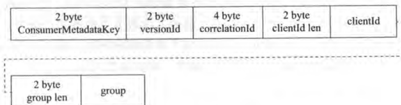
图 4-27 ConsumerMetadataRequest 二进制数据组成
