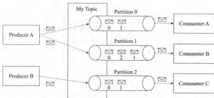
图 2-4 消息发送的简易流程
