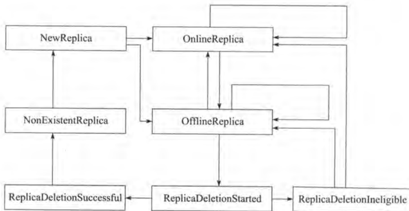
图 5-5 分区副本状态的生命周期
