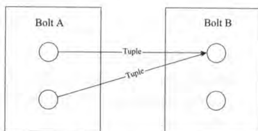
图 9-5 Global Grouping
