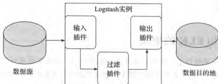
图 9-7 Logstash 功能
