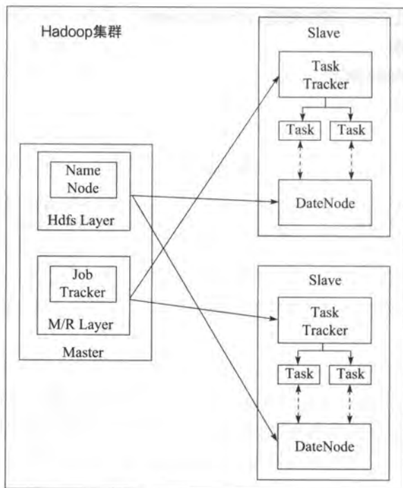
图 9-9 HDFS+MapReduce
