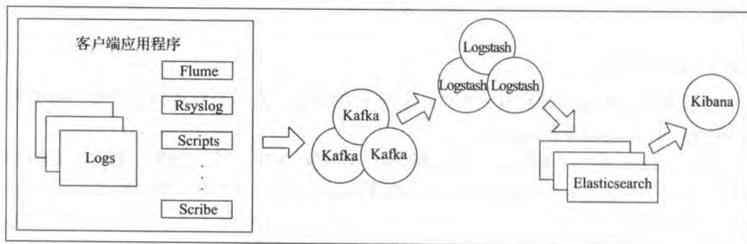
图 9-8 Kafka+ELK
