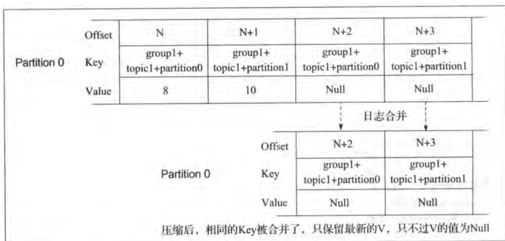
图 4-14 Compact 策略
