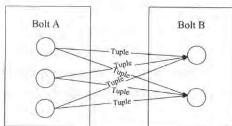
图 9-4 All Grouping
