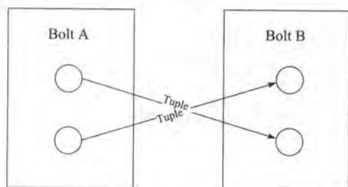
图 9-2 Shuffle Grouping
