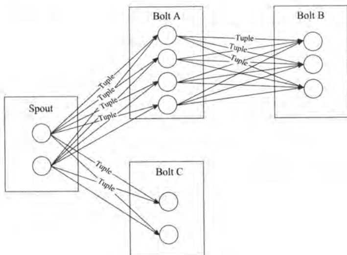
图 9-1 Storm 的 Topology
