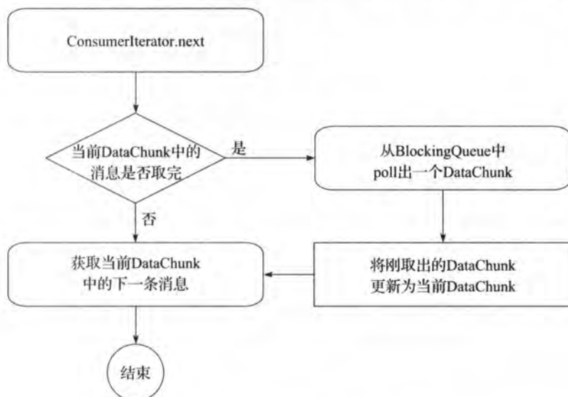
图 8-4 ConsumerIterator 的实现原理
