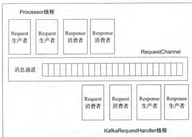
图 4-2 简单的生产者和消费者模型
