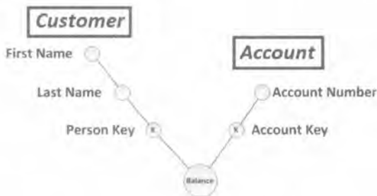
图 8-3 太阳模型（一个事实，两个维度）
