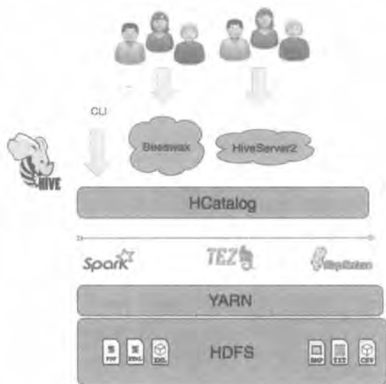
图 3-1 Hive 组件
