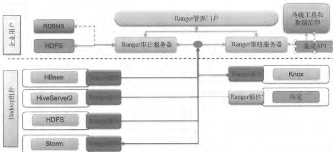
图 10-1 Ranger 架构
