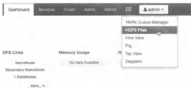
图 7-1 HDFS 视图
