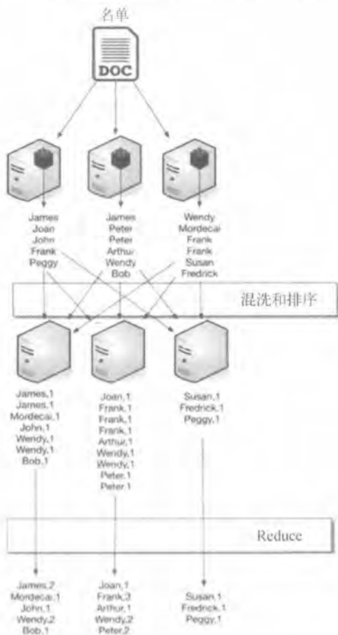
图 1-8 Reduce 阶段
