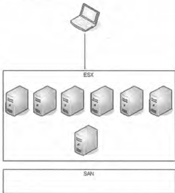
图 1-2 虚拟化架构
