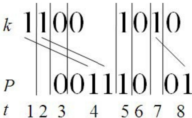
图9-25 手算方案
