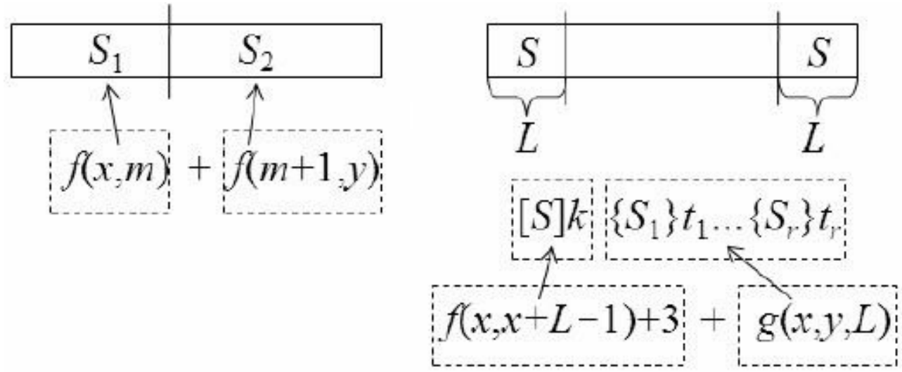
图12-64 连接
