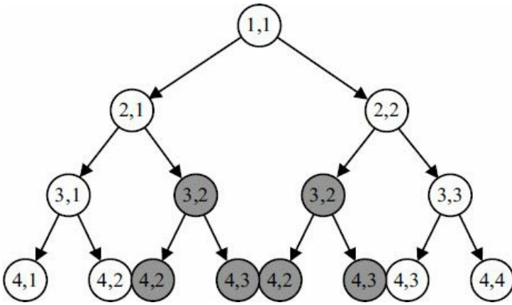
图9-2 重叠子问题
