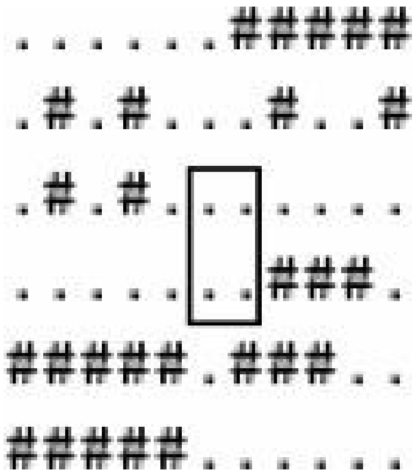
图12-82 最优解
