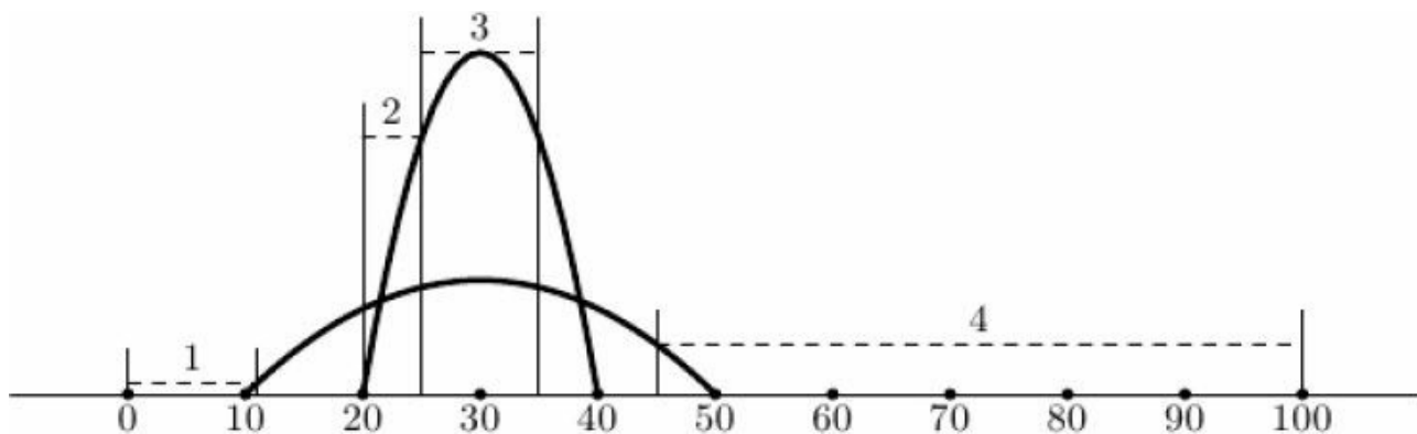
图12-30 导弹飞行轨迹
