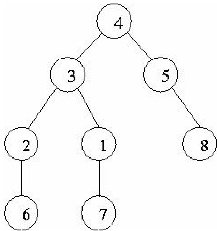
图6-29 树重建
