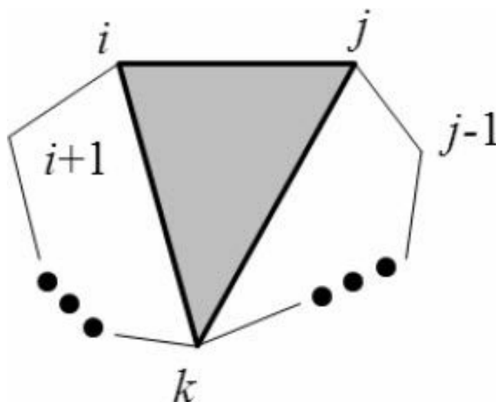
图9-10 定义的子多边形
