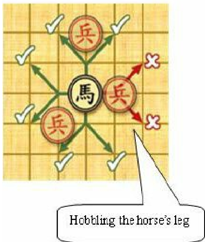
图4-4 “蹩马腿”情况
