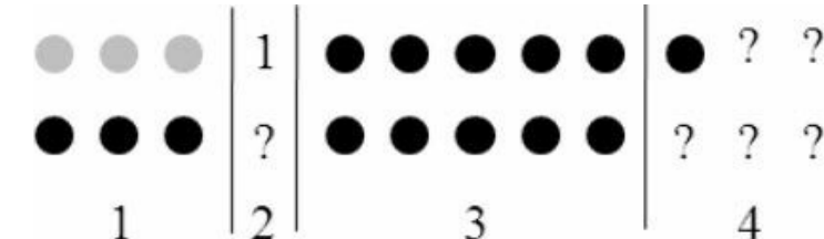
图8-25 赛程安排的4个阶段
