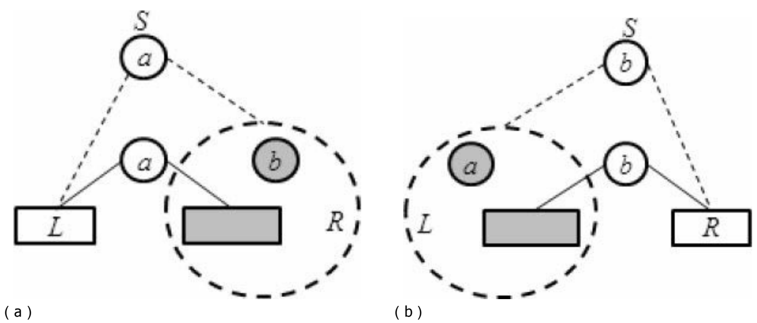
图12-19 merge操作
