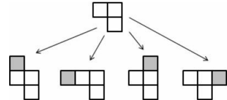
图7-23 回溯法求解
