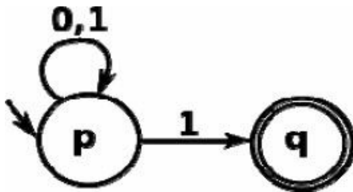
图12-2 NFA示例
