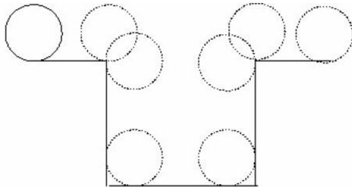
图12-50 更复杂的轮子滚动状态
