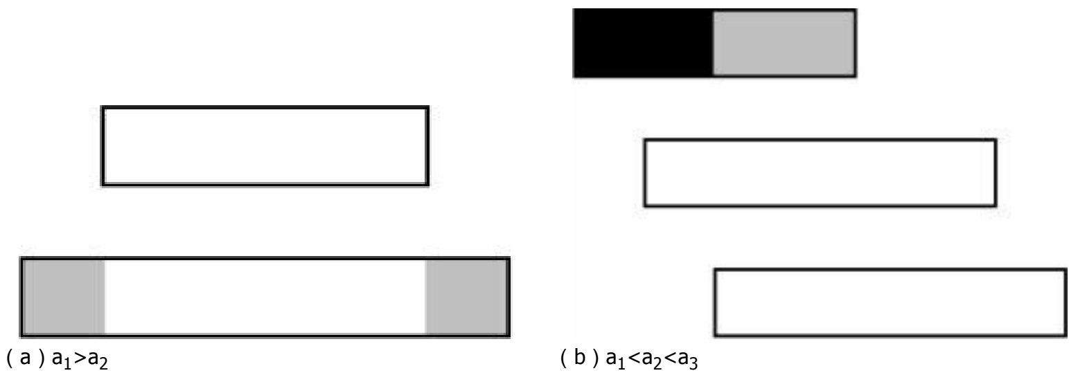
图8-7 贪心策略图示
