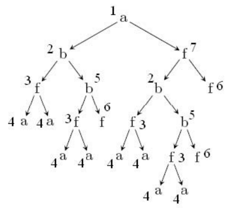
图11-4 子树编写
