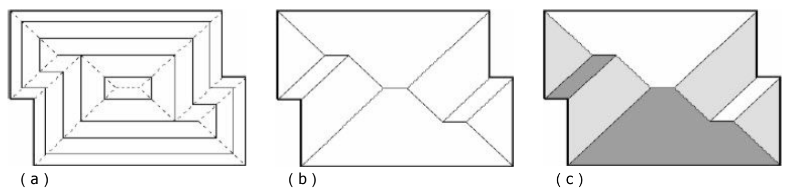
图12-79 屋顶
