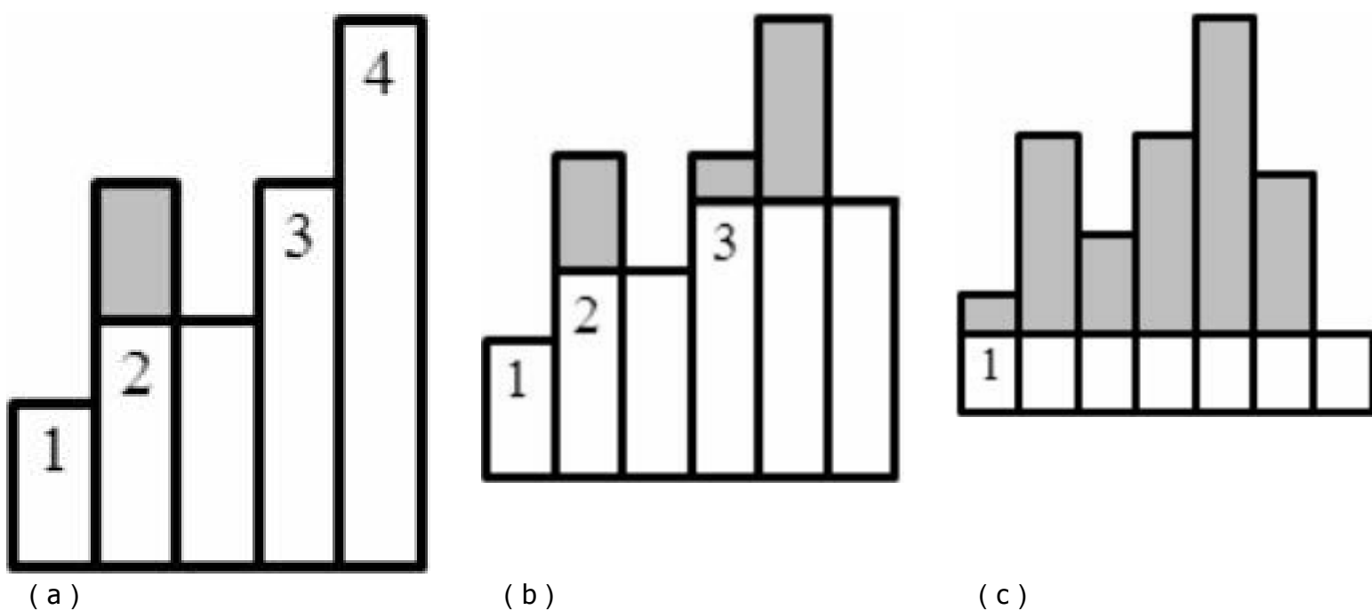
图8-29 移动当前列
