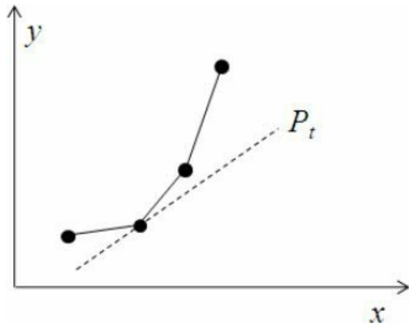
图8-18 最优点 P_t
