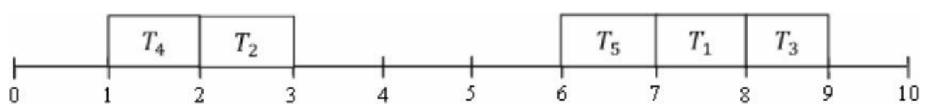
图8-33 最优解
