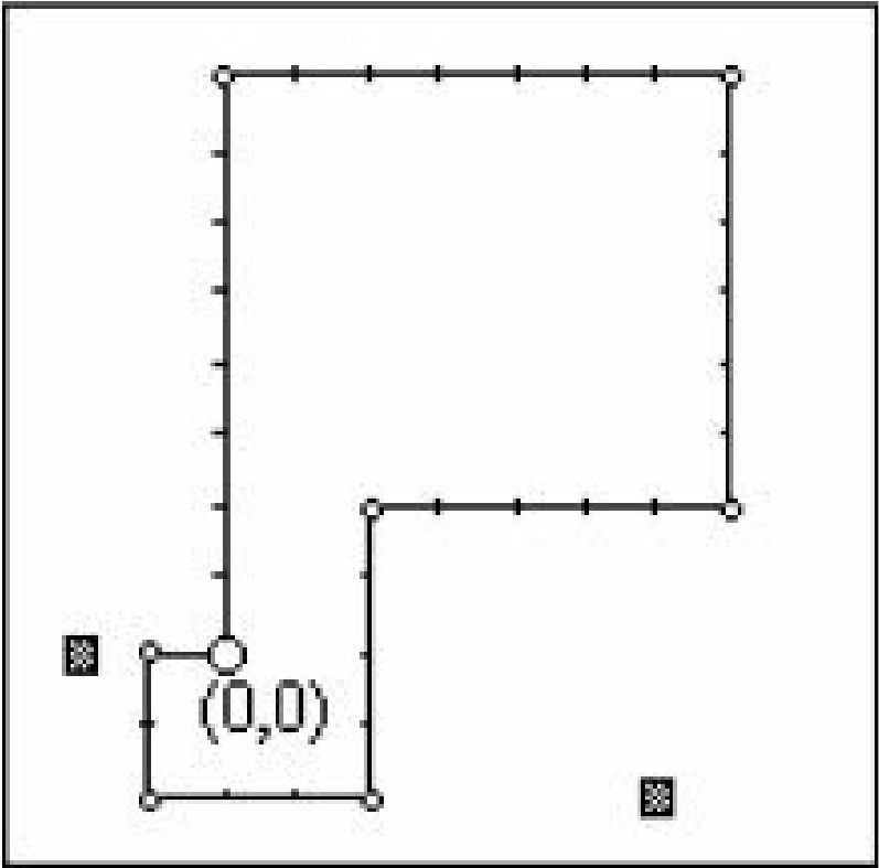
图7-25 黄金图形示意图
