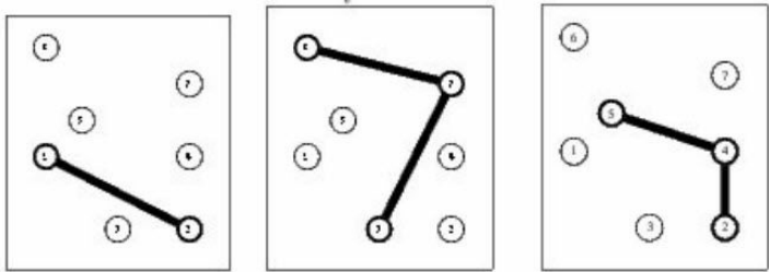
图11-6 3个套餐
