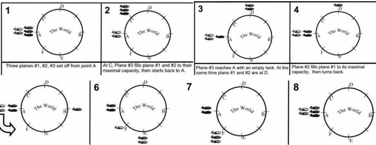
图10-22 飞机环球问题示意图
