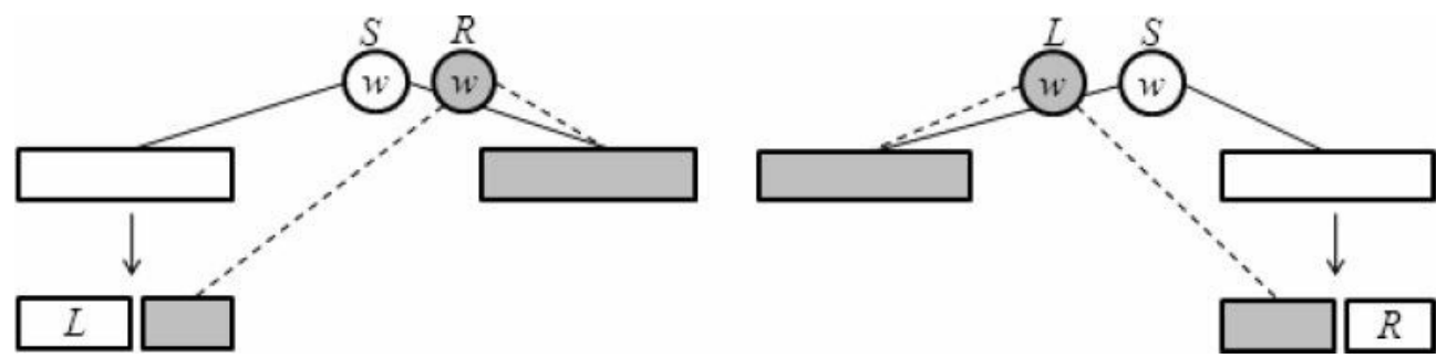
图12-18 split操作
