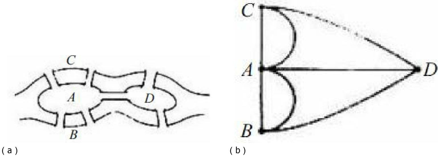
图6-15 七桥问题
