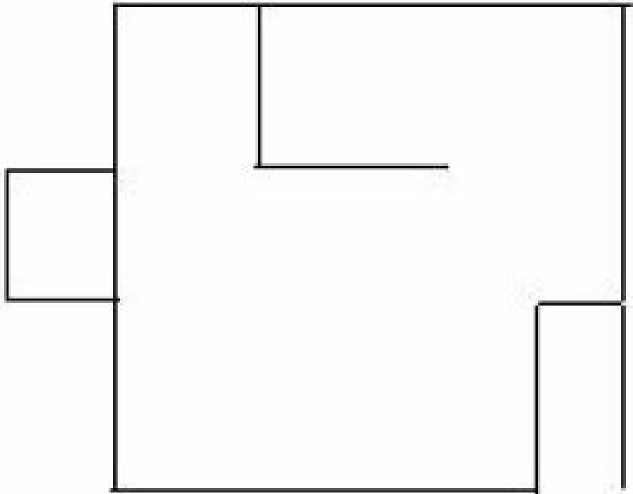
图12-76 图形示例
