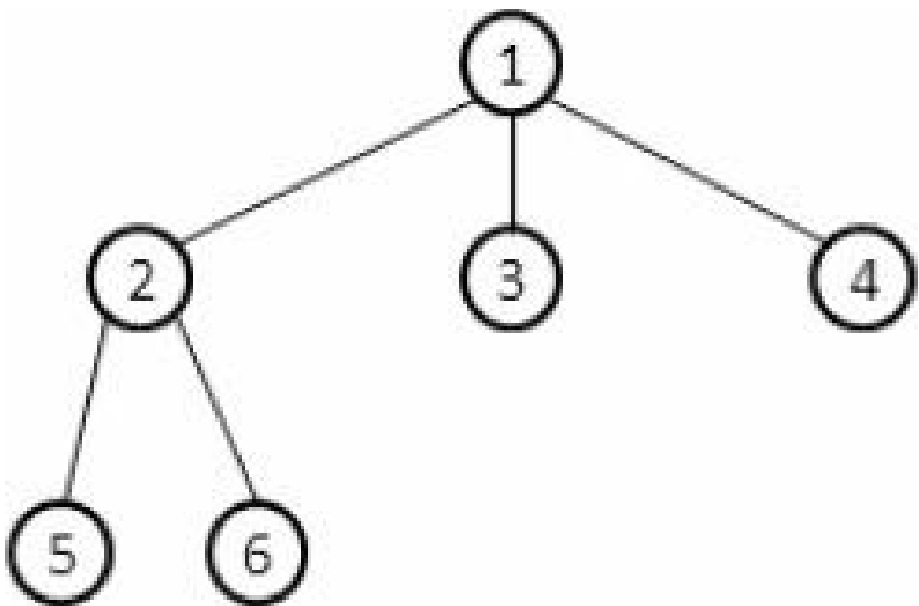
图12-10 欧拉序列
