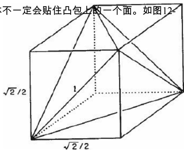
图12-60 正四面体
