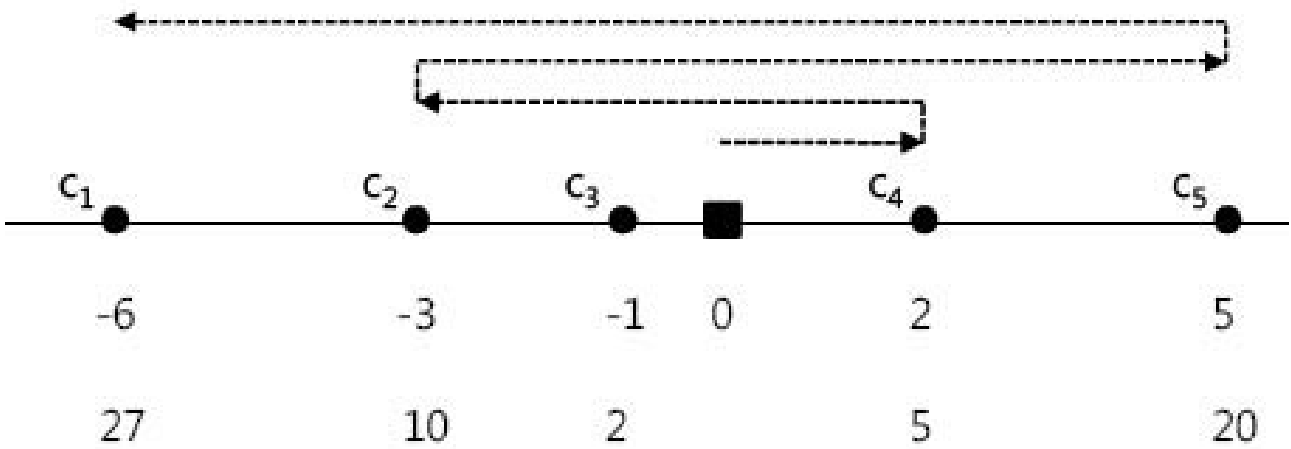
图9-28 送餐路线
