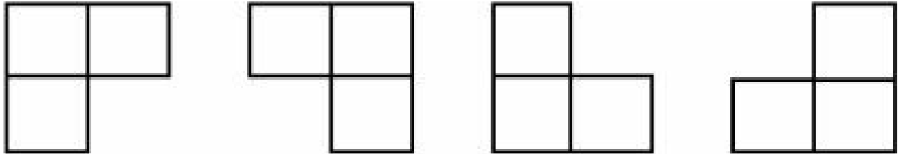
图8-3 L型牌
