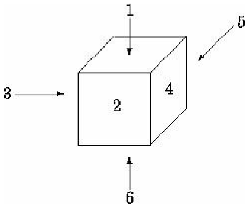
图4-7 骰子涂色
