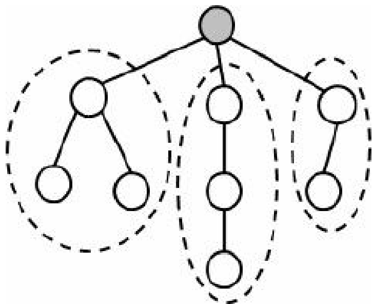
图12-8 分治算法
