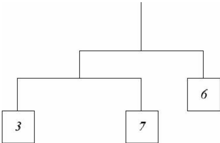
图6-23 修改天平
