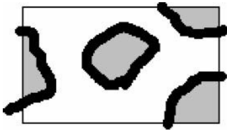
图6-18 战场示意图
