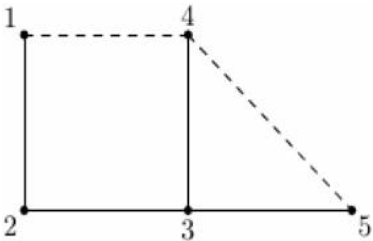
图11-23 “王国的道路图”问题示意图
