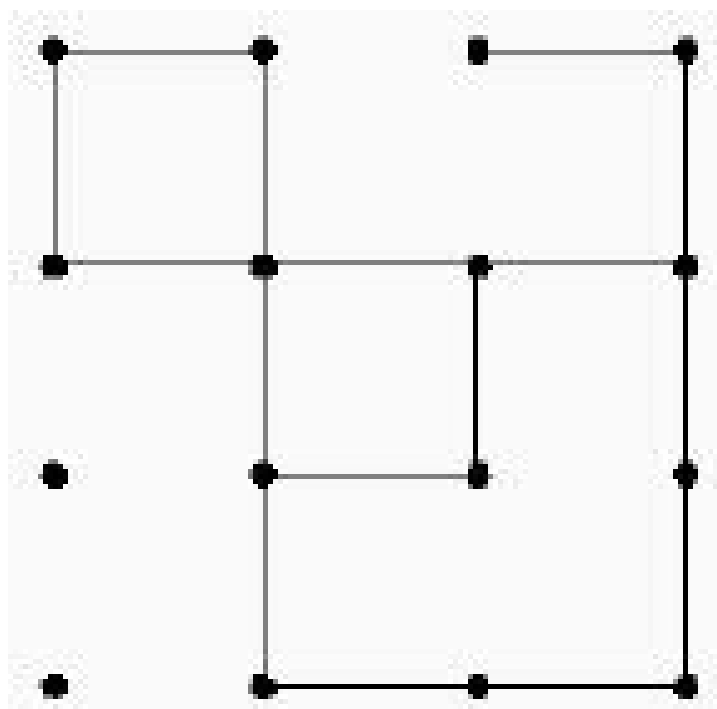
图4-5 正方形
