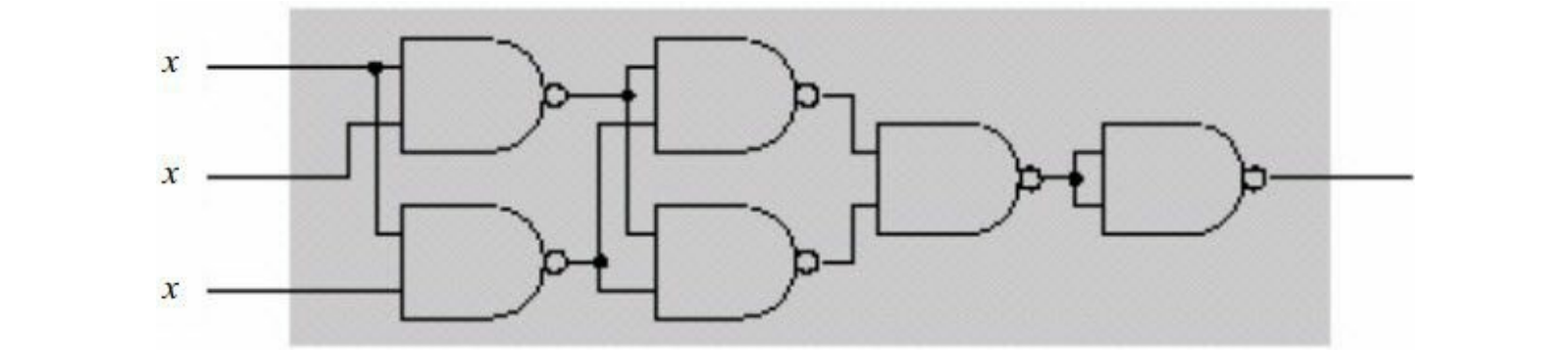
图8-22 与非门输入电路
