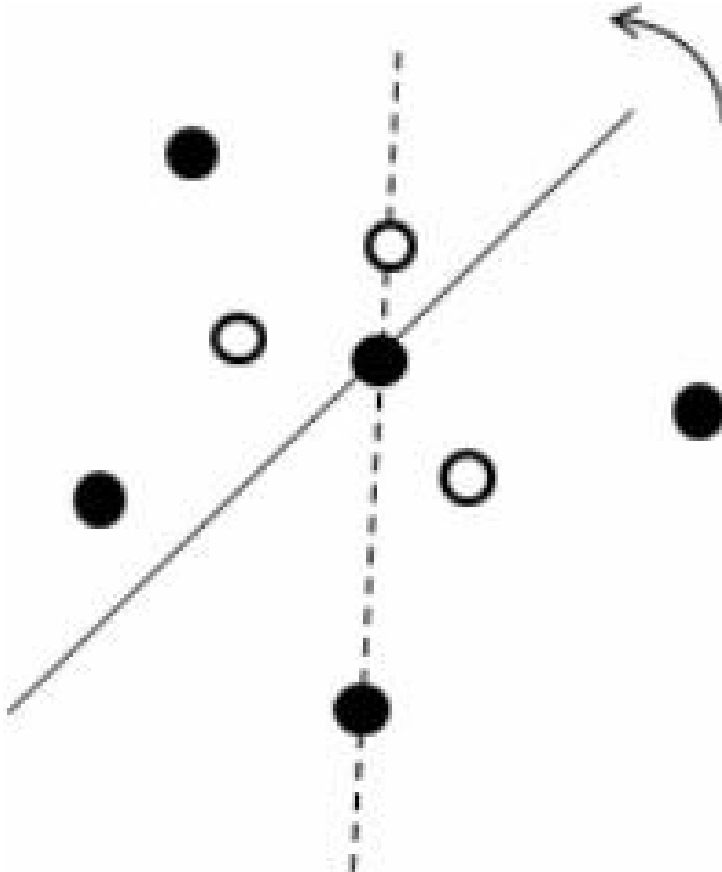
图8-12 枚举基准点
