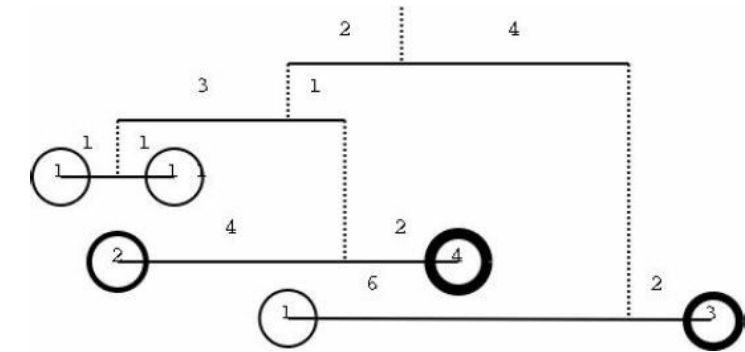
图6-6 正确输出
