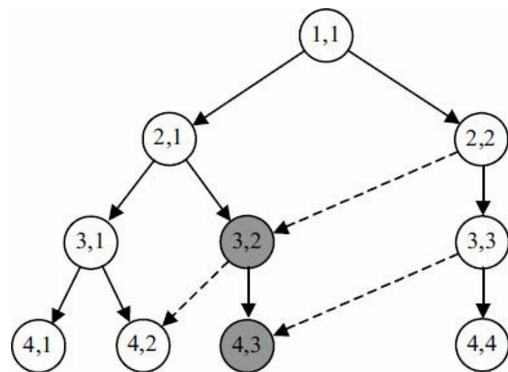
图9-3 记忆化搜索
