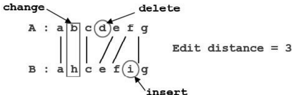
图9-36 编辑距离
