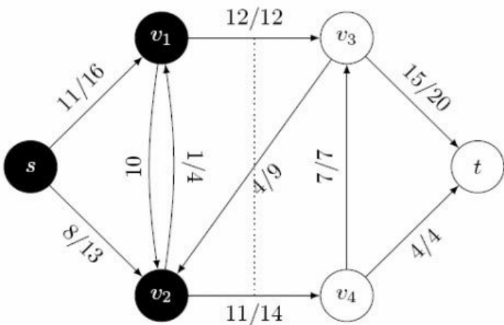
图11-11 网络中的割
