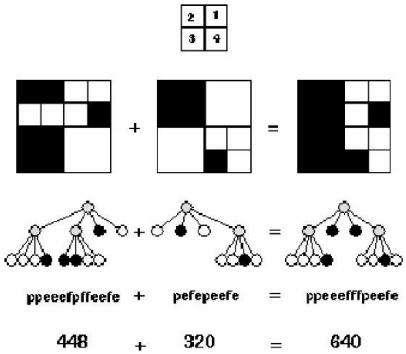
图6-8 四分树
