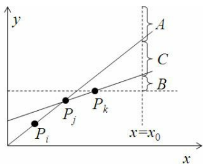
图8-16 平均值问题示意图
