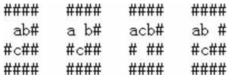
图7-18 4种移动方式
