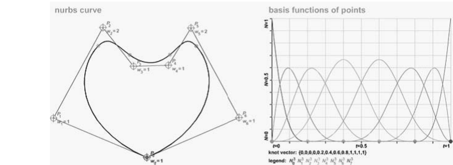
图12-56 NURBS曲线
