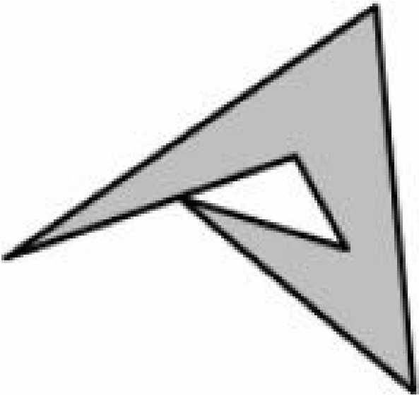
图12-25 非规范相交
