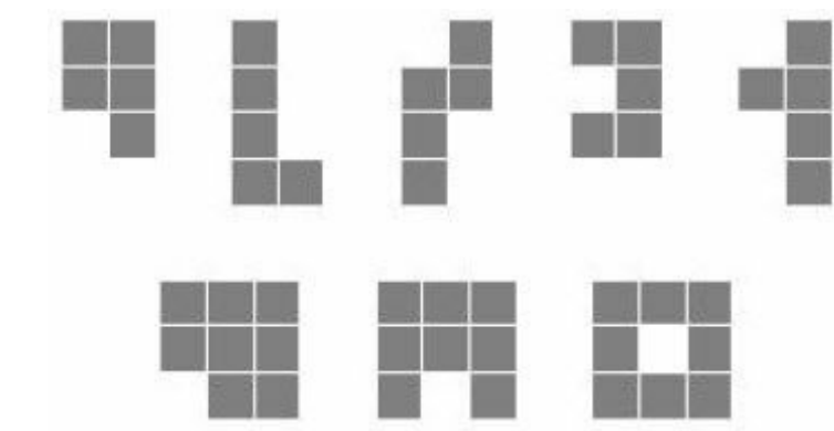
图7-22 网格动物例题示意图
