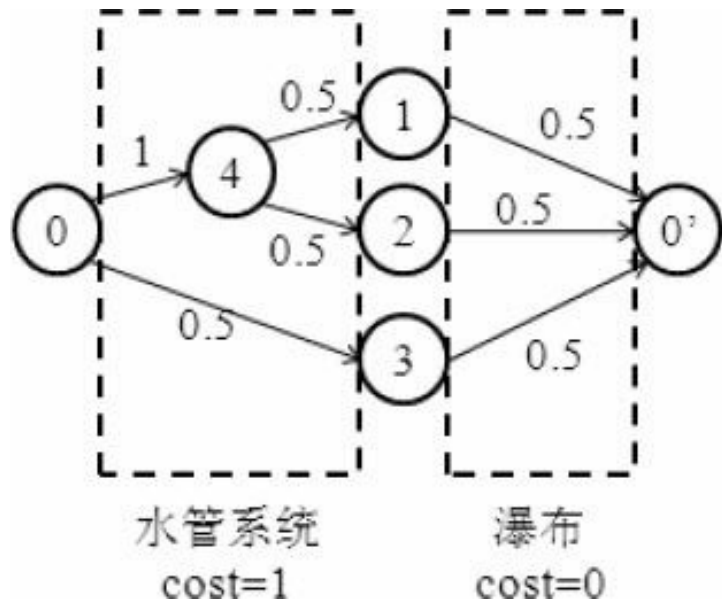
图12-38 唯一可行解
