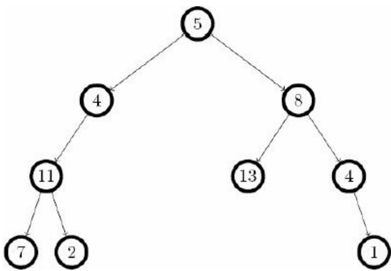
图6-3 一棵二叉树
