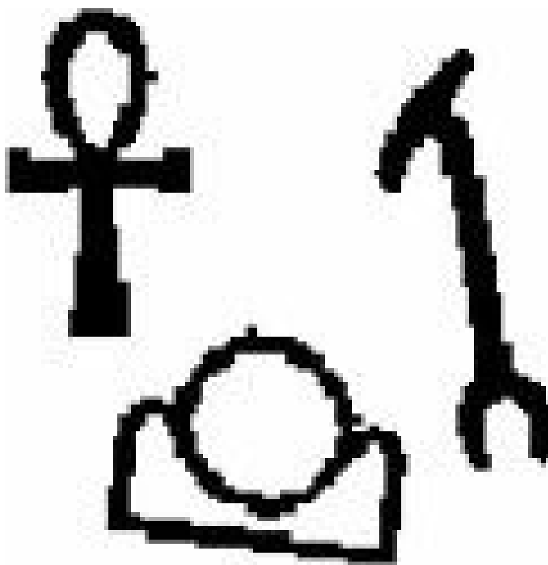
图6-11 输出AKW
