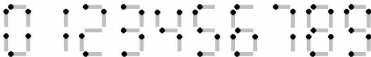
图9-17 火柴数字
