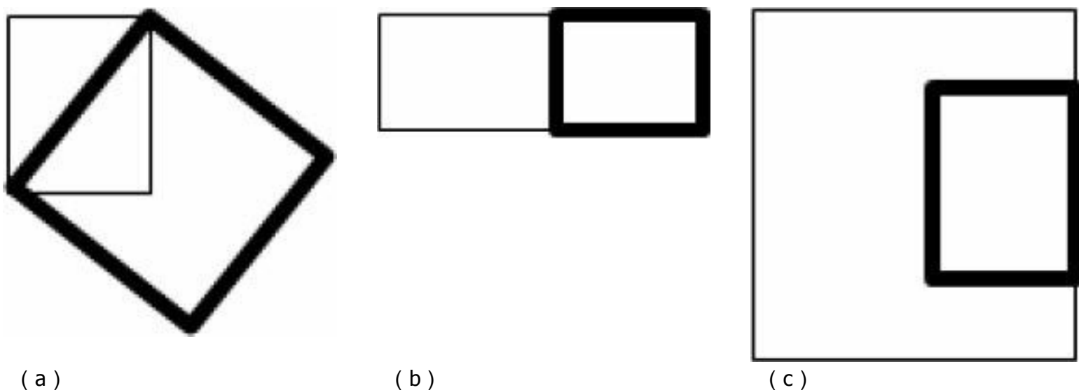
图12-21 多边形相交问题分析
