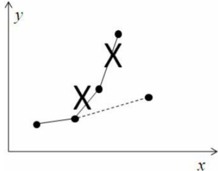
图8-17 下凸点
