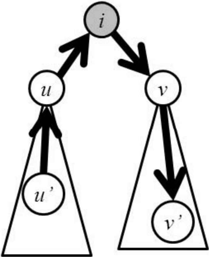
图9-21 最长链
