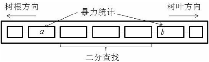
图12-34 实现update ( a，b，v，res1，res2 )
