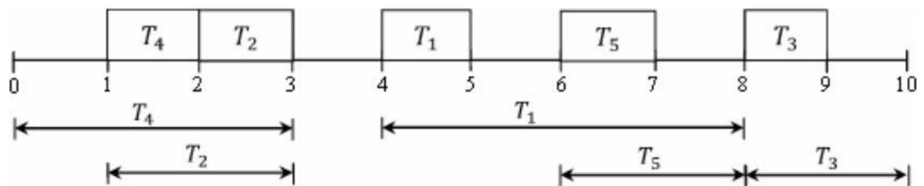
图8-32 5条线段范围
