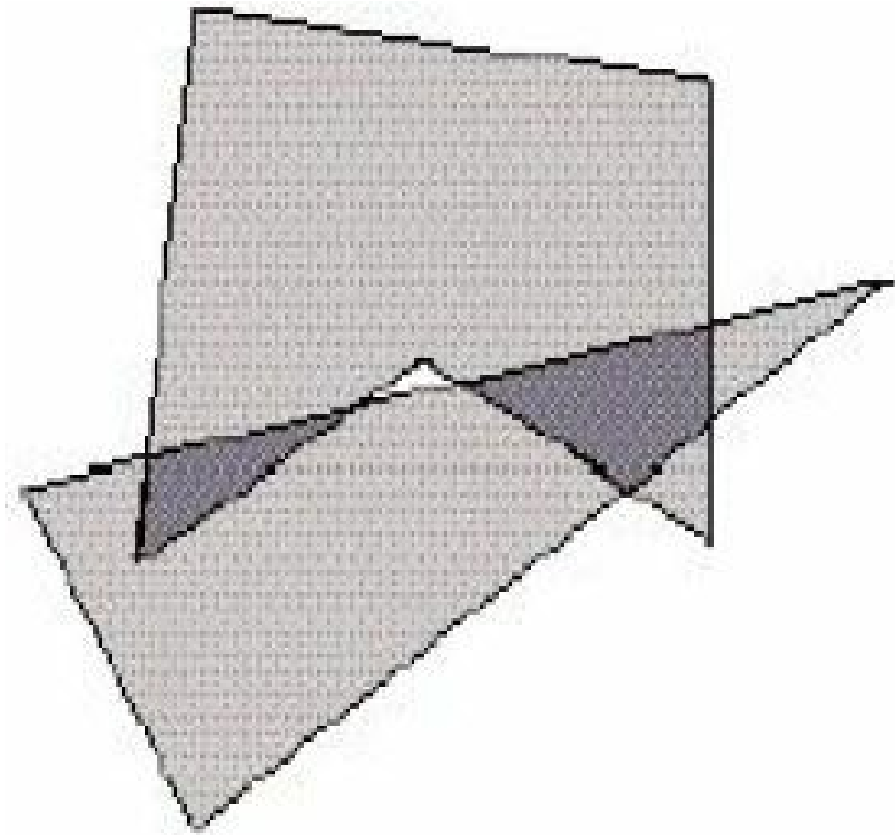
图12-20 多边形相交
