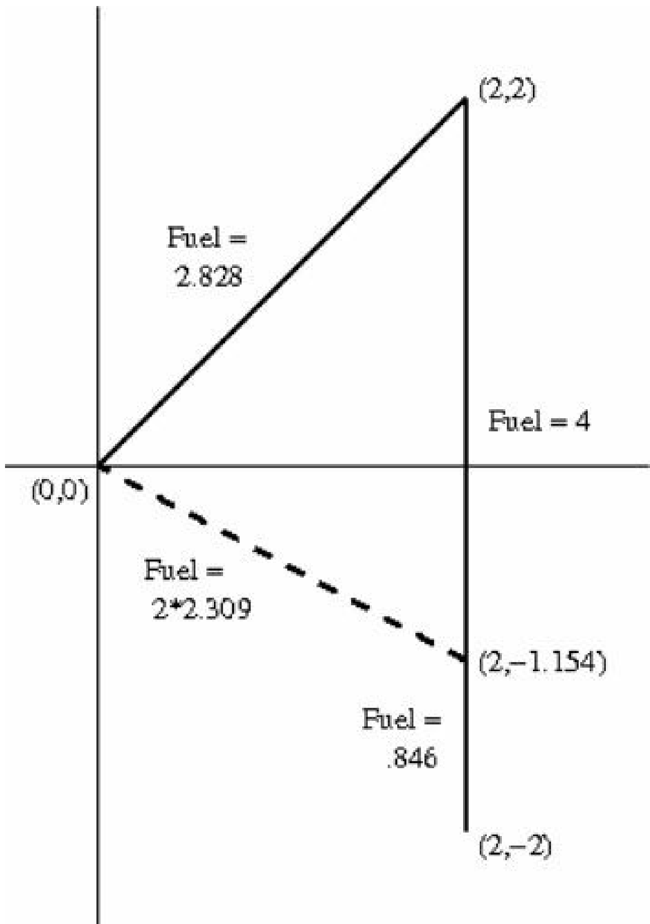
图11-24 行驶路线
