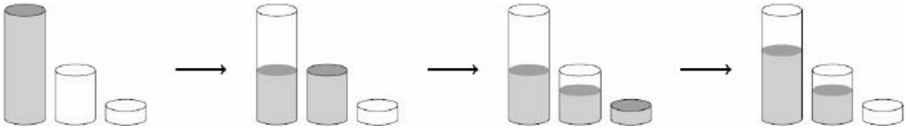
图7-15 倒水问题：一种方法是 (6,0,0) \rightarrow (3,3,0) \rightarrow (3,2,1) \rightarrow (4,2,0)
