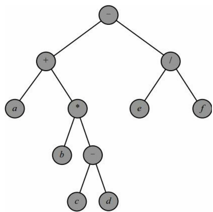
图11-2 表达式树
