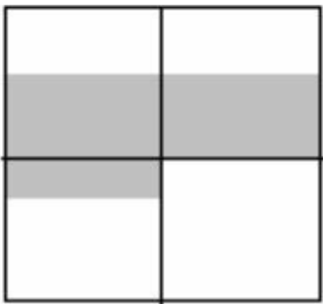
图8-20 k 小时的情况
