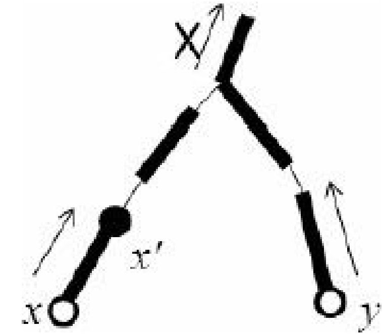
图12-33 查询操作
