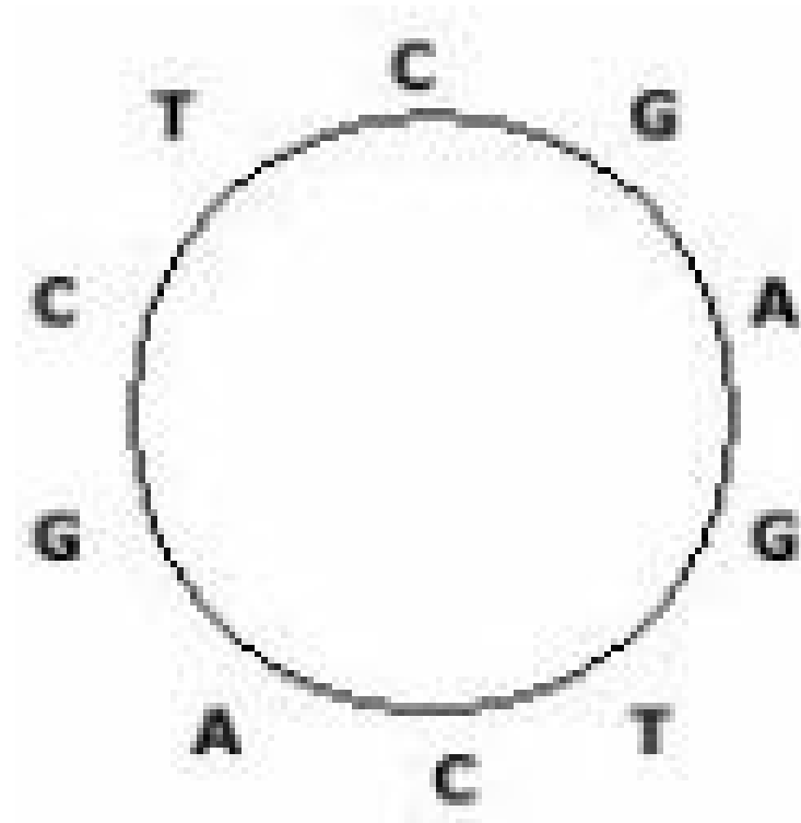
图3-4 环状串
