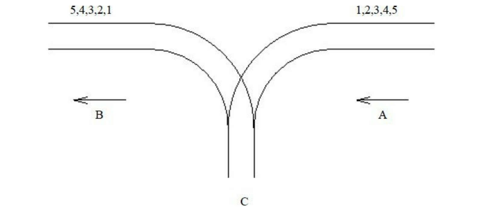
图6-1 铁轨
