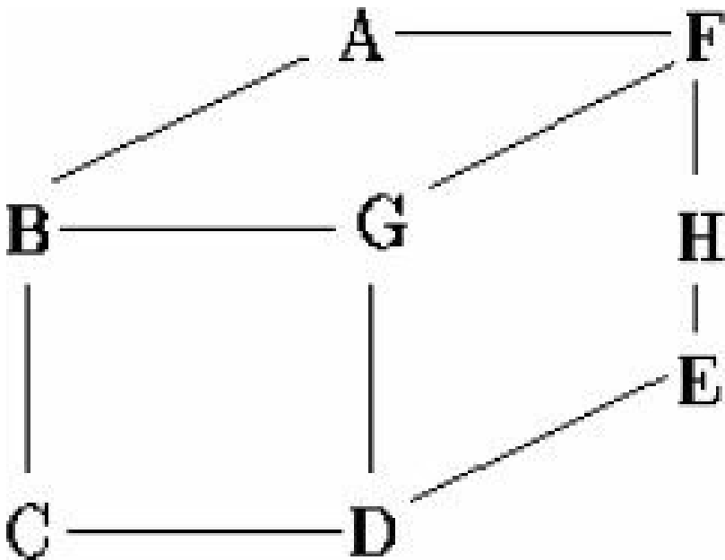
图7-7 图G
