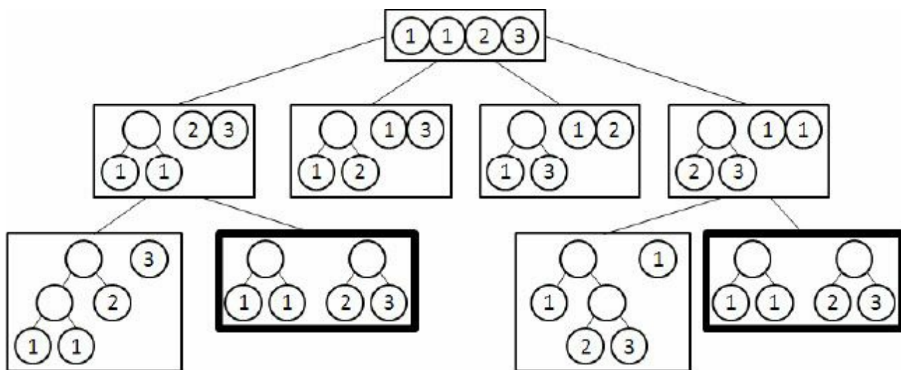
图7-13 解答树
