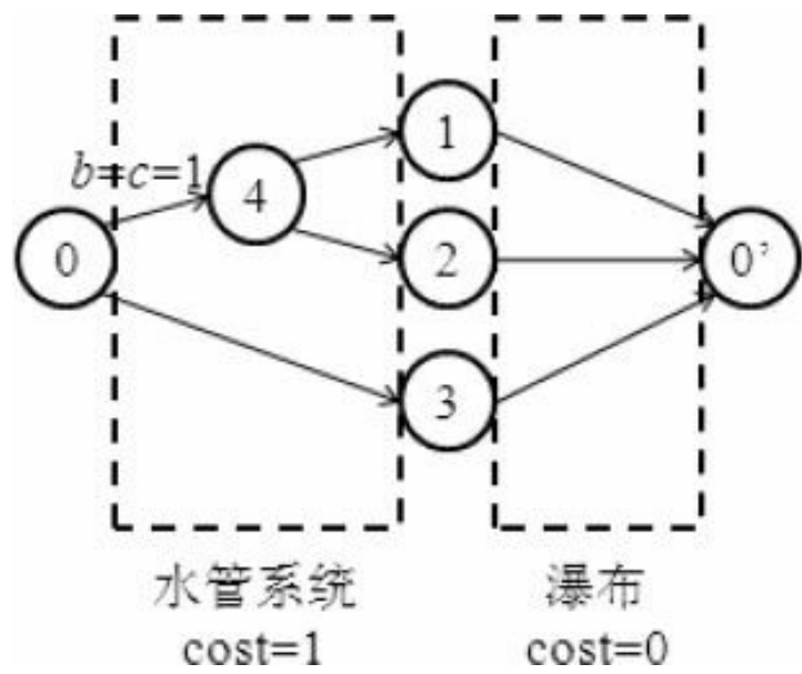
图12-37 瀑布弧
