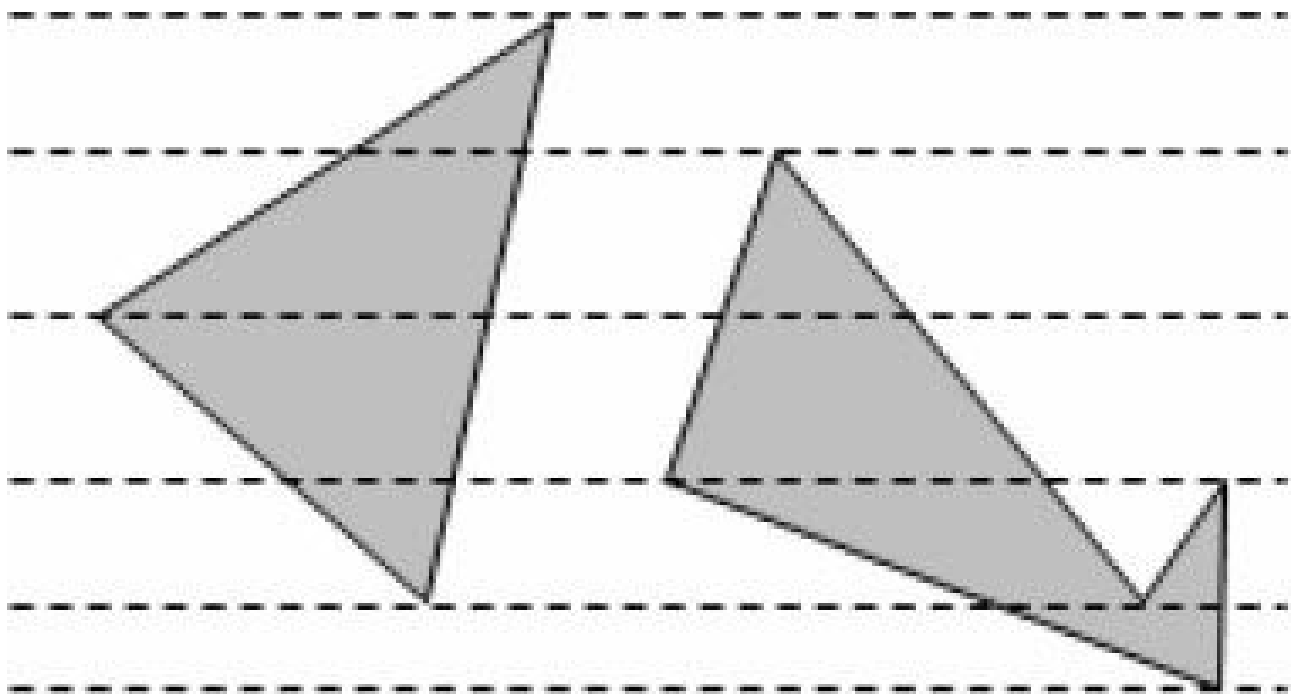
图12-47 水平线划分出的梯形或三角形
