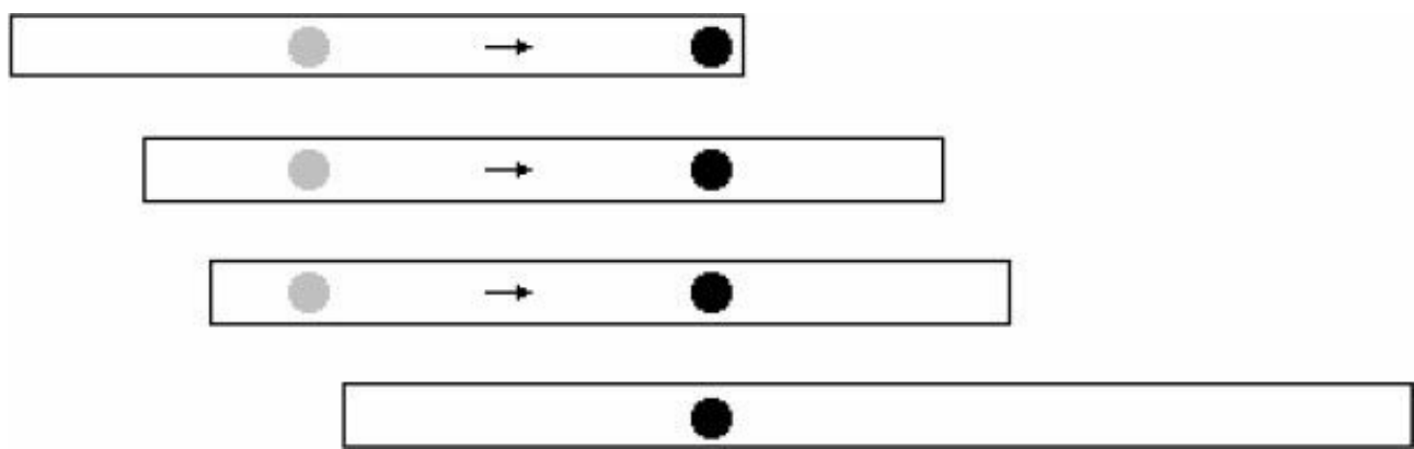
图8-8 贪心策略
