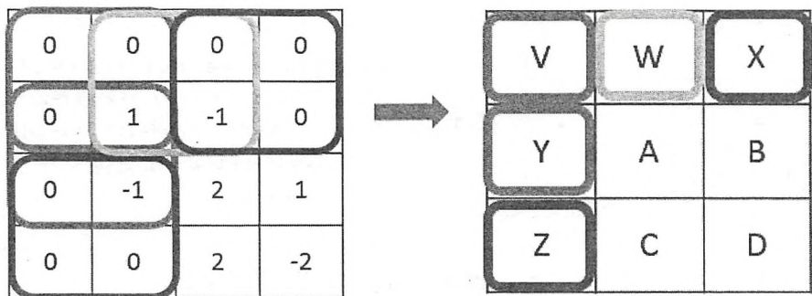
图 6-11 使用了全 0 填充（zero-padding）的卷积层前向传播示意图 ①
