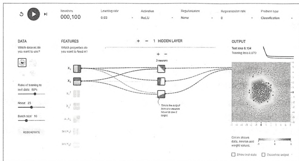
图 4-4 使用非线性模型解决线性不可分问题的效果
