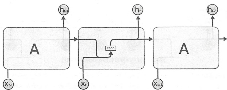
图 8-4 使用单层全连接神经网络作为循环体的循环神经网络结构图 ③
