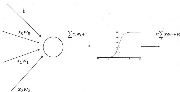
图 4-5 加入偏置项和激活函数的神经元结构示意图
