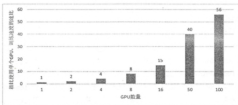
图 10-8 训练速度随着 GPU 数量增加的变化趋势，此数据来自谷歌官方的测试结果 ①
