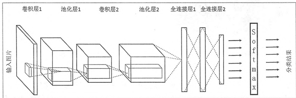
图 6-7 用于图像分类问题的一种卷积神经网络架构图
