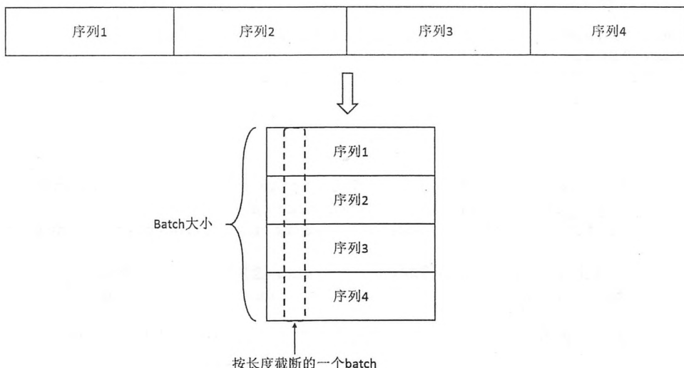
图 8-11 将一个长序列分成 batch 并截断的操作示意图
