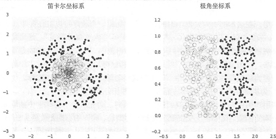
图 1-1 不同的数据表达对使用直线划分不同颜色结点的难度影响
