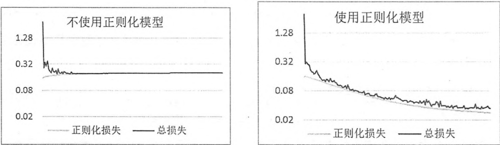
图 5-7 正则化损失值和总损失的变化趋势
