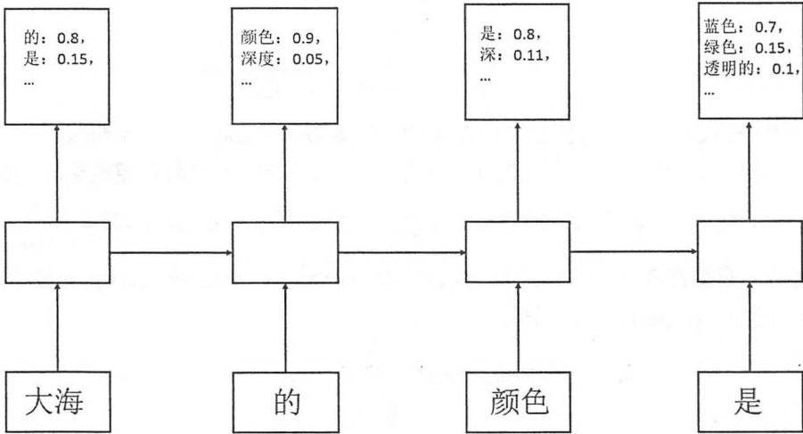
图 8-10 使用循环神经网络实现自然语言建模示意图
