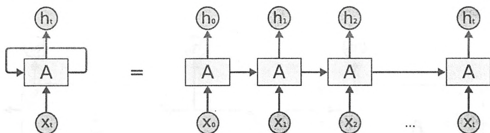
图 8-2 循环神经网络按时间展开后的结构
