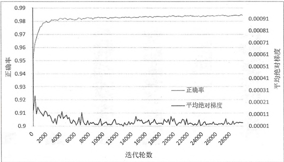
图 5-4 使用了所有优化方法的模型正确率与平均绝对梯度在不同迭代轮数时的变化趋势
