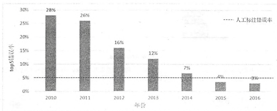
图 1-7 历年 ILSVRC 图像分类比赛最佳算法的错误率
