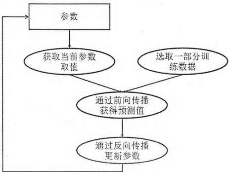
图 10-1 深度学习模型训练流程图
