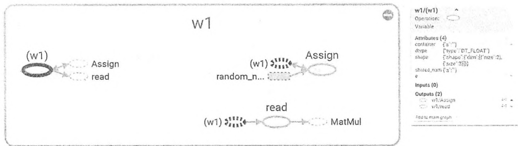
图 3-7 神经网络前向传播样例中变量 w1 相关部分的计算图可视化结果 ①
