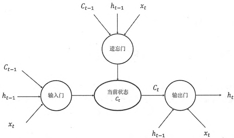
图 8-6 LSTM 单元结构示意图
