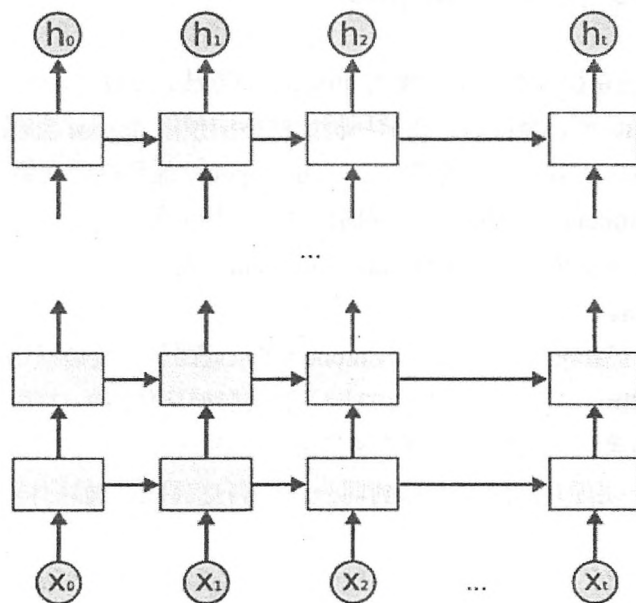
图 8-8 深层循环神经网络结构示意图
