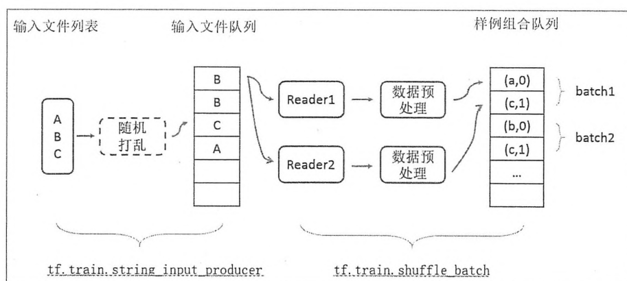
图 7-15 输入数据处理流程示意图
