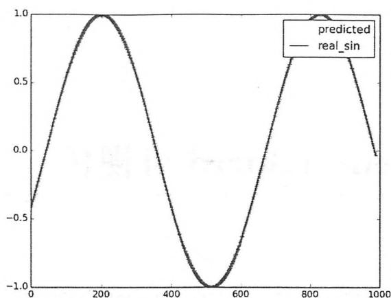
图 8-13 通过循环神经网络预测 sin 函数得到的结果
