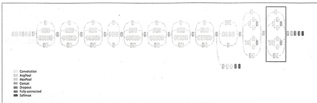
图 6-17 Inception-v3 模型架构图
