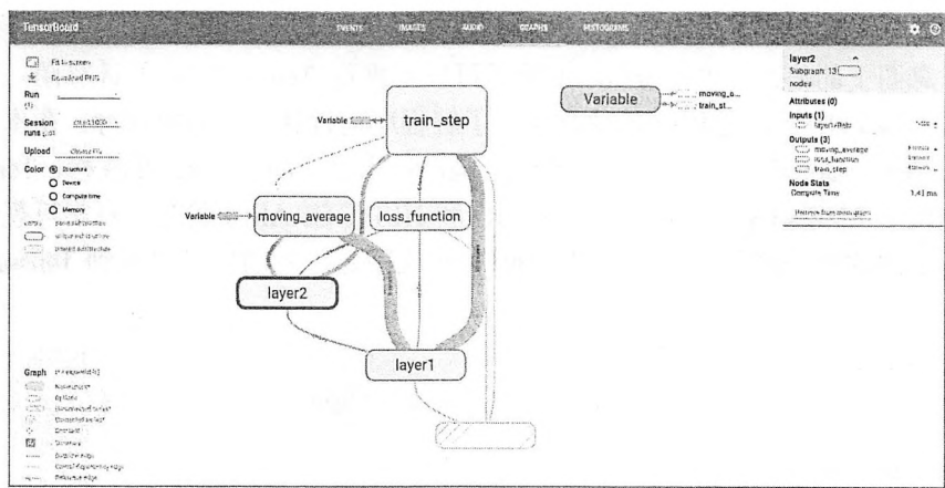
图 9-14 TensorFlow 命名空间在 TensorBoard 可视化效果图上的信息卡片
