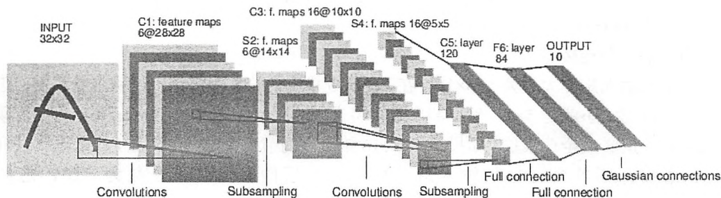
图 6-15 LeNet-5 模型结构图 ②
