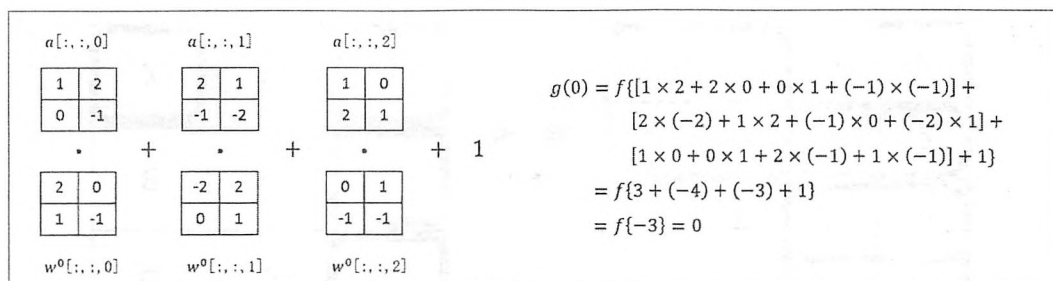
图 6-9 使用过滤器计算 g(0) 取值的过程示意图
