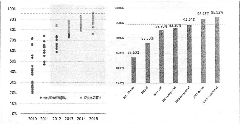
图 6-5 不同算法在 ImageNet ILSVRC2012 图像分类数据集上的正确率
