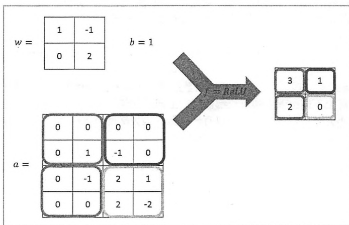
图 6-13 卷积层前向传播过程样例图
