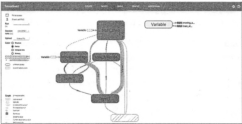
图 9-13 使用了 GPU 的 TensorFlow 计算图的可视化结果
