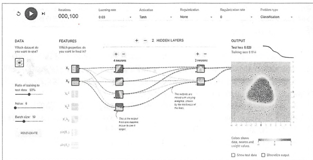
图 3-3 TensorFlow 游乐场训练 100 轮之后的截图
