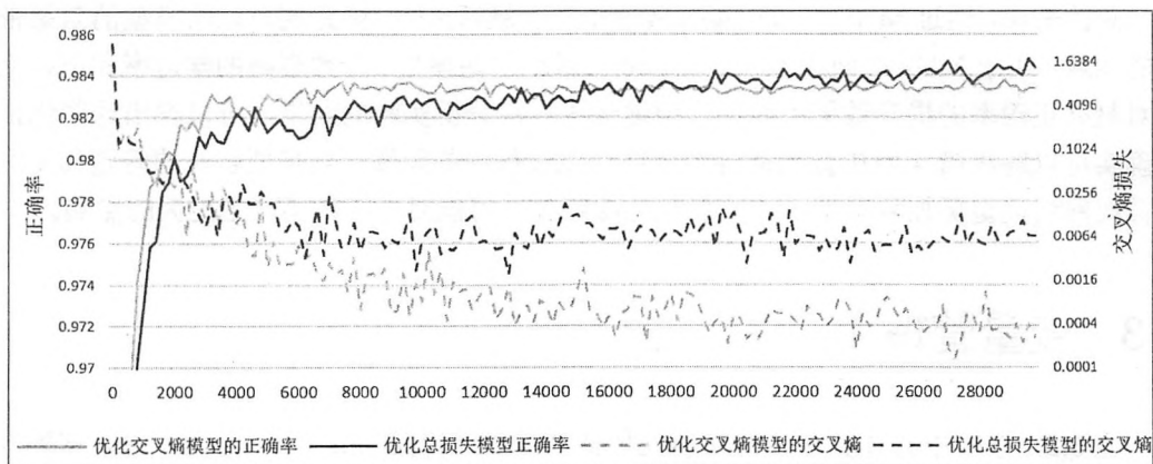
图 5-6 不同模型在不同迭代轮数时交叉熵和正确率的关系
