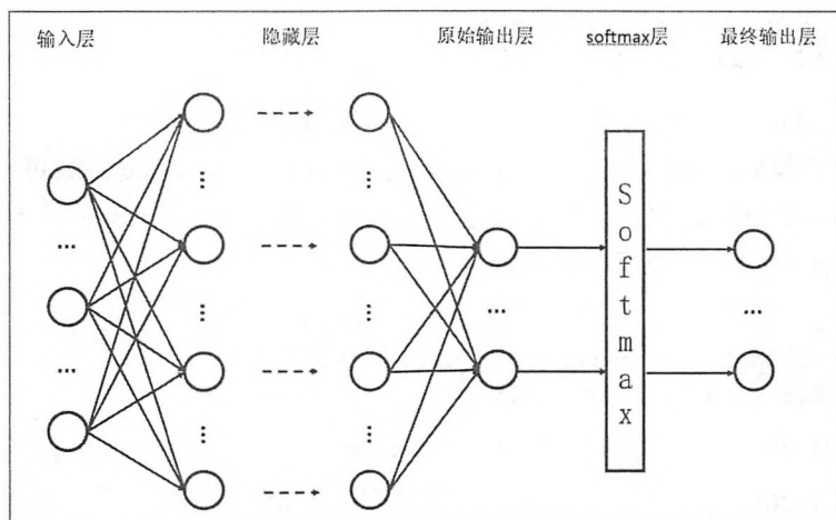
图 4-10 通过 Softmax 层将神经网络输出变成一个概率分布
