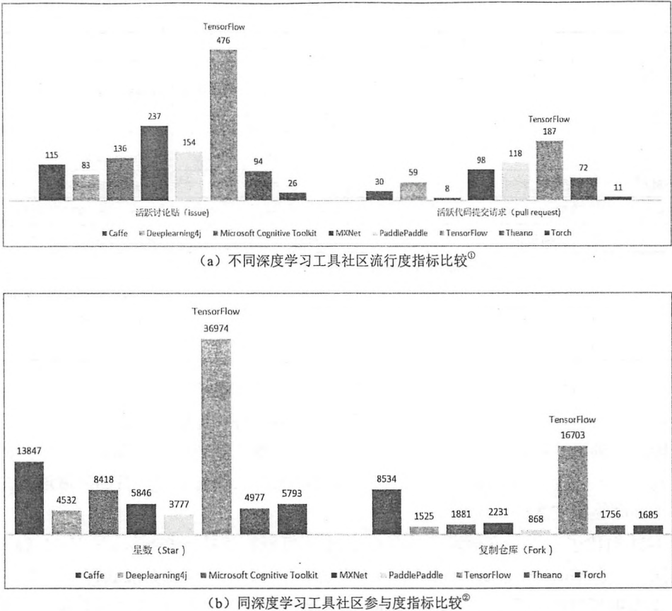
图 1-11 不同深度学习工具在 GitHub 上活跃程度对比图
