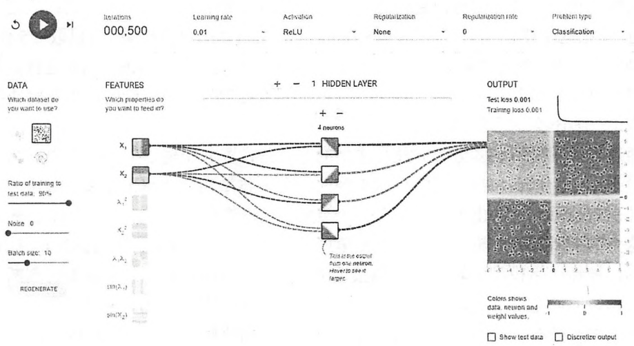
图 4-9 使用深层神经网络解决异或问题
