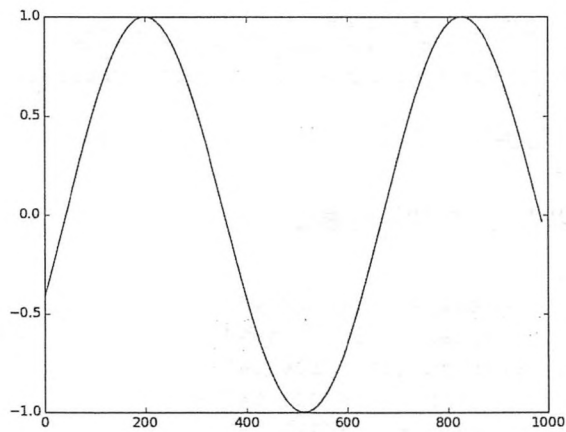
图 8-12 sin 函数曲线
