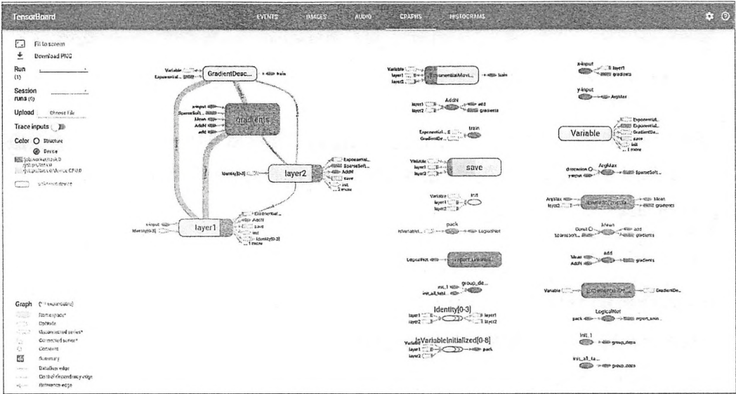
图 10-9 通过 TensorBoard 可视化的分布式 TensorFlow 计算图
