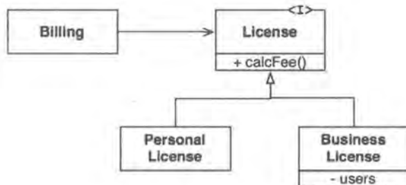
图 9.1: License 类与其衍生类，体现了 LSP 原则
