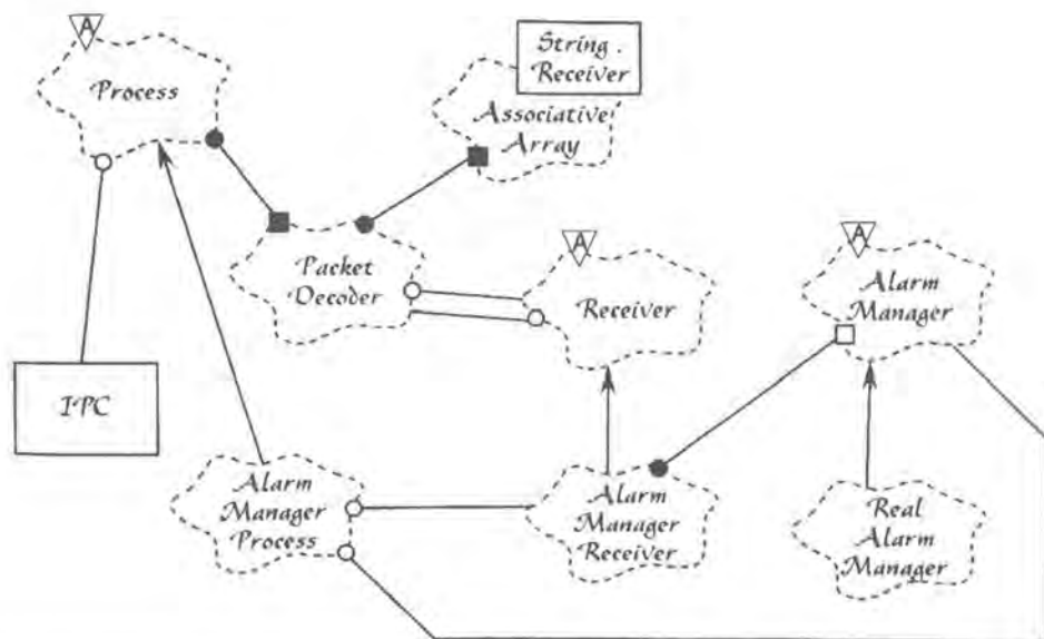
图 A.9: Booch 图
