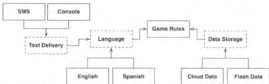
图 25.3: 修正后的设计图
