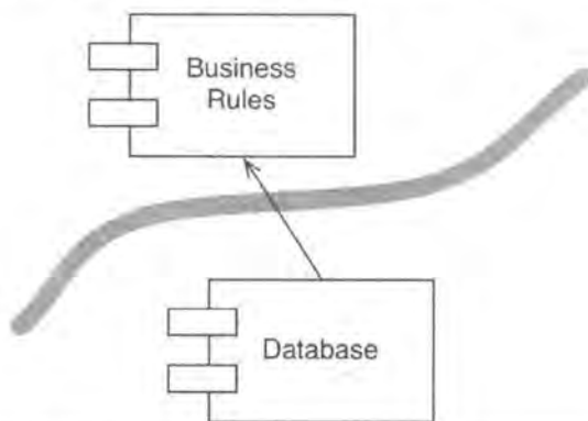
图 17.3: 业务逻辑组件与数据库组件
