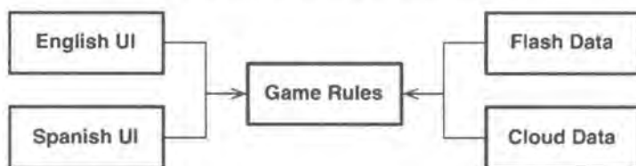
图 25.2: 遵循依赖关系规则的设计
