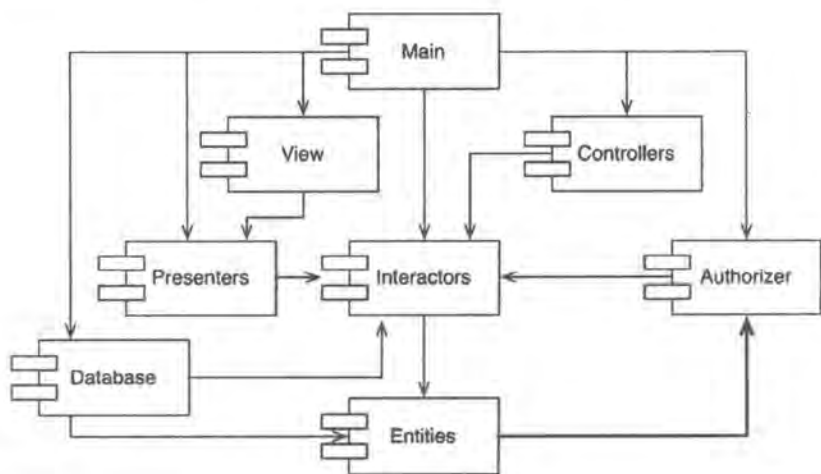
图 14.2: 循环依赖
