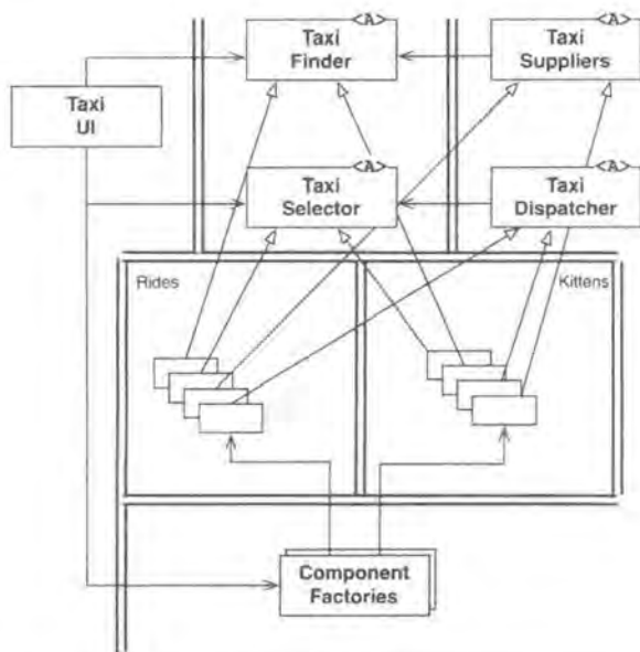
图 27.2：采用面向对象的方法来处理横跨型变更
