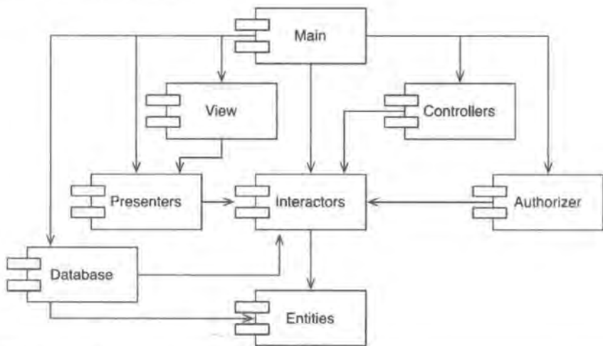
图 14.1: 典型的组件结构图
