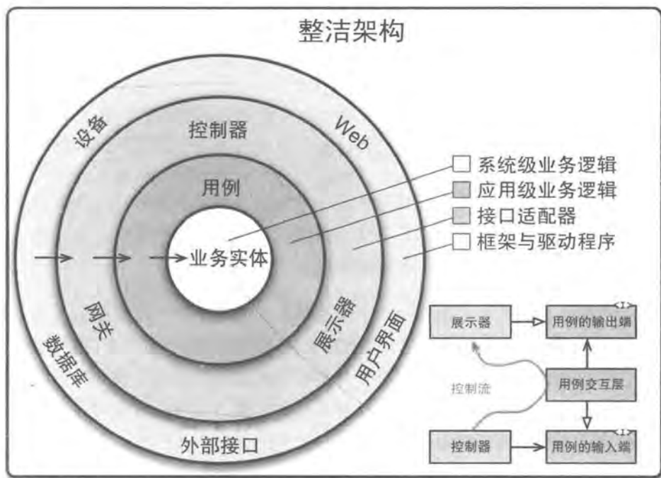
图 22.1: 整洁架构
