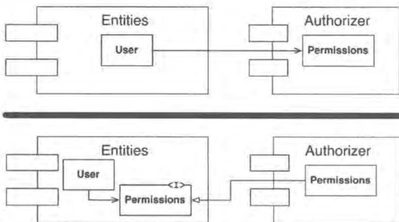
图 14.3: 将 Entities 与 Authorizer 之间的依赖关系反转
