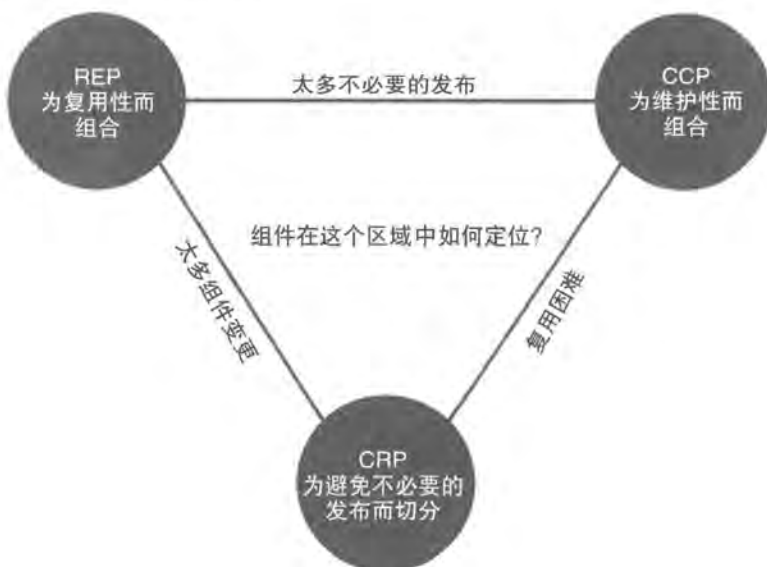
图 13.1: 组件聚合原则的张力图
