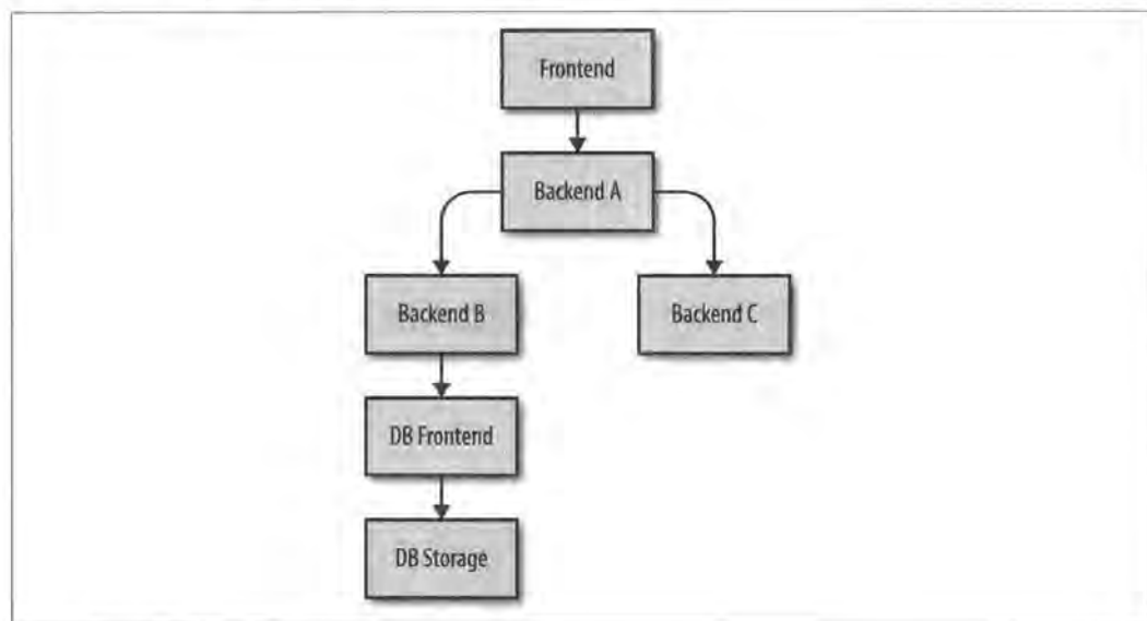
图21-2：某个依赖栈
