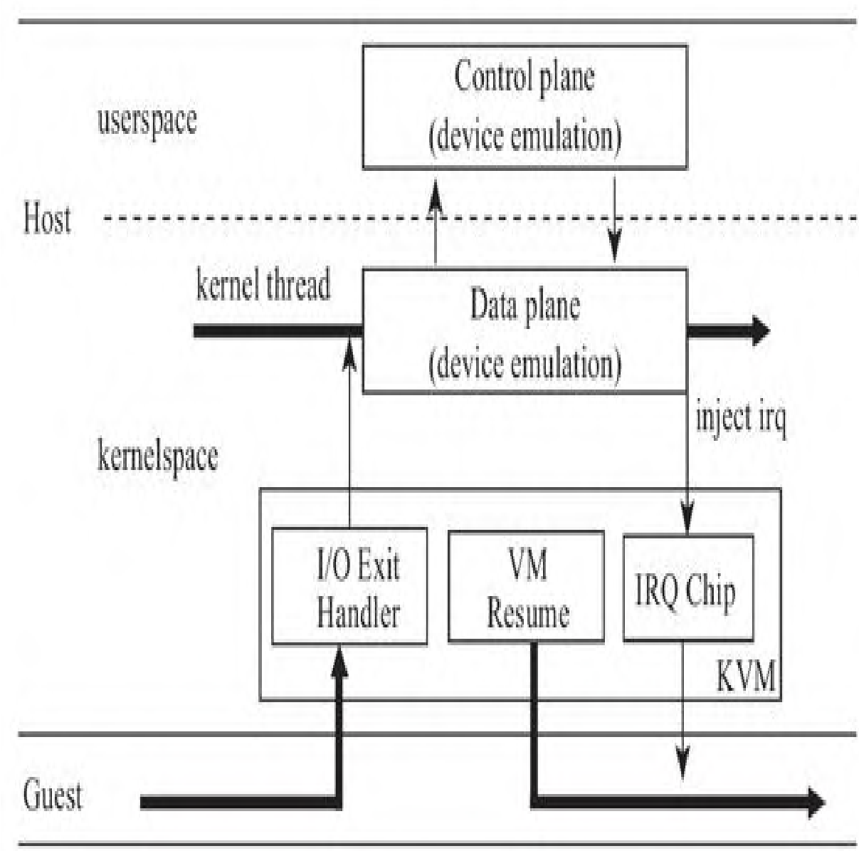
图4-2 Vhost虚拟化
