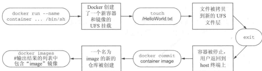
图 7-1 从容器中构建镜像
