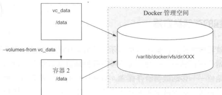
图 4-8 容器 2 复制了 vc_data 的存储卷句柄
