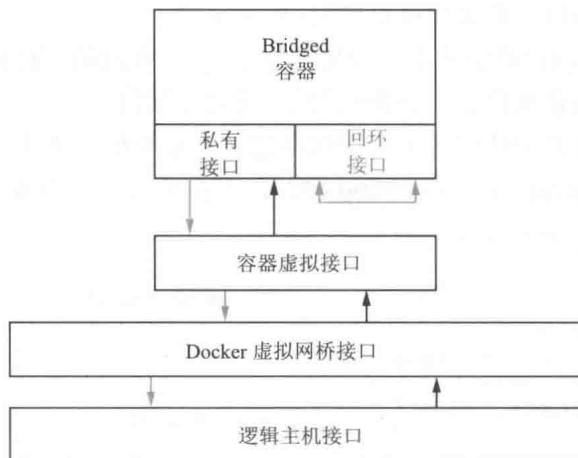
图 5-8 Bridged 容器的入站流量
