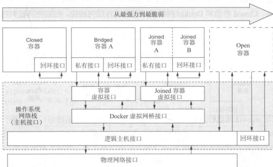
图 5-5 四种网络容器原理以及它们与 Docker 网络拓扑结构的关系
