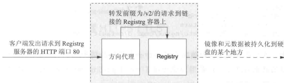
图 10-3 在客户端和 Registry 之间插入一个反向代理
