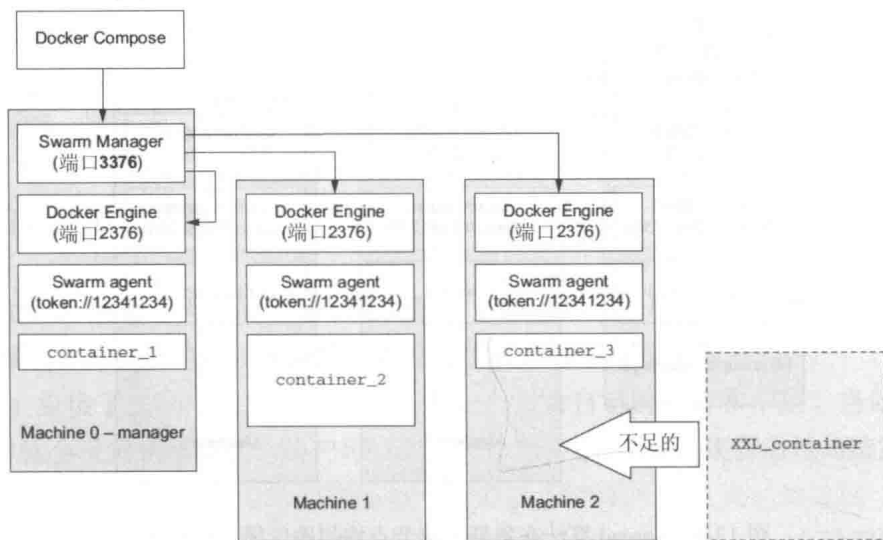
图 12-7 由于分布不均，新的容器无法被调度
