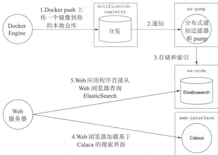
图 11-1 数据流经由四个容器组成的通知 Registry 的示例
