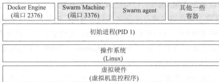
图 12-3 Swarm、Swarm manager 和另外的程序，这些程序都是在一个典型的虚拟机里的 Docker 引擎的 Docker 容器里运行的
