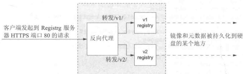
图 10-5 基于请求的 Registry API 版本进行客户端路由
