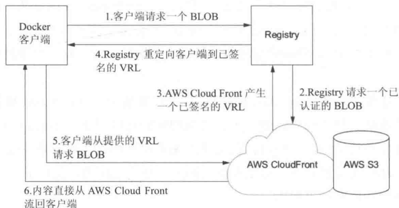
图 10-8 用 AWS CloudFront 存储中间件消除流处理 BLOB 流量
