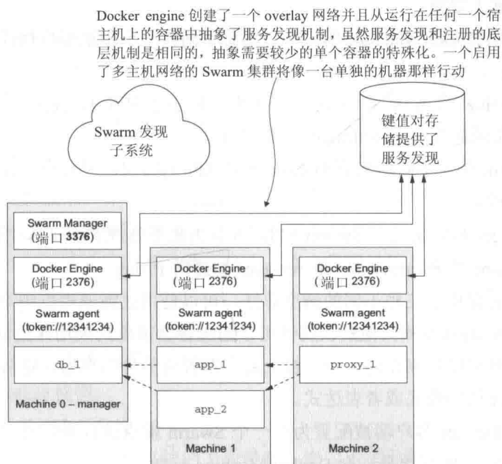
图 12-13 Docker 引擎上面的 Swarm 和多主机网络使得集群可以作为一个单独的机器，而容器充当网络中的平等成员
