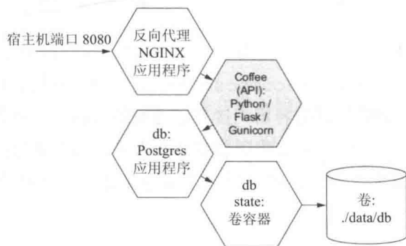
图 11-2 本章示例环境的服务和服务依赖
