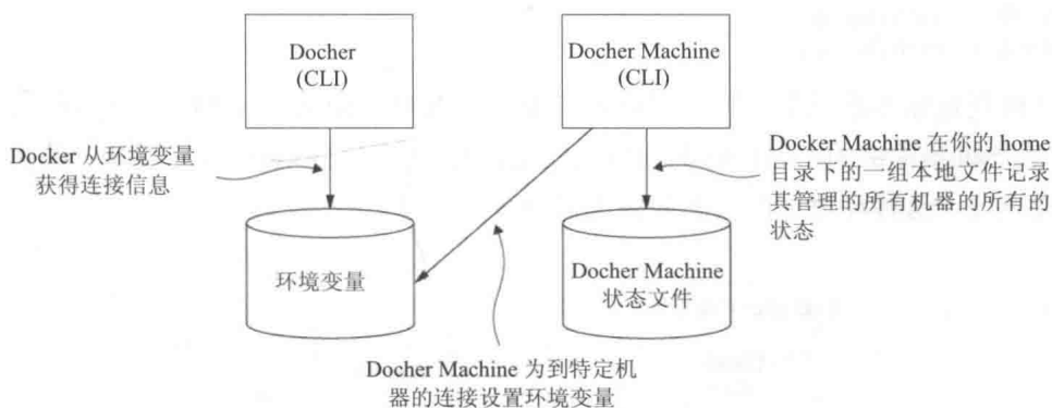
图 12-1 docker、docker-machine 和相关的状态资源之间的关系
