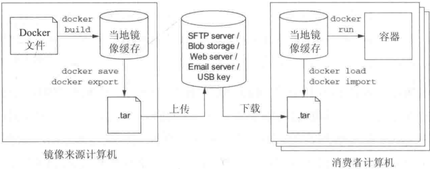
图 9-7 生产者、传输和消费者之间的一个典型的手动分发工作流程
