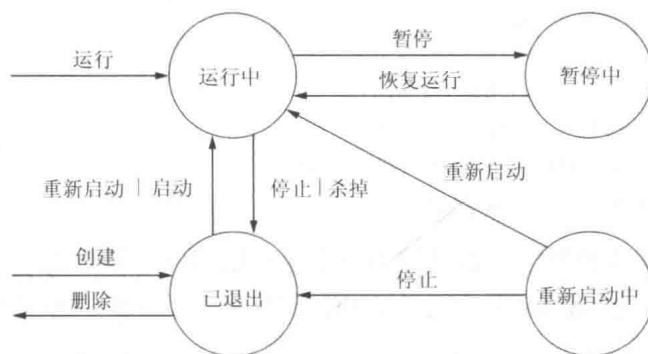
图 2-3 Docker 容器的状态转移图
