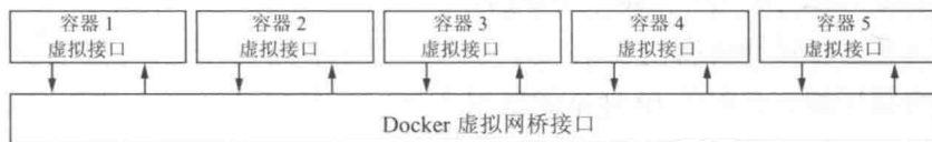
图 5-9 连接在同一个 Docker 网桥（docker 0）上的五个容器
