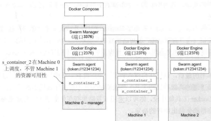
图 12-10 随机调度算法选择机器仅考虑概率
