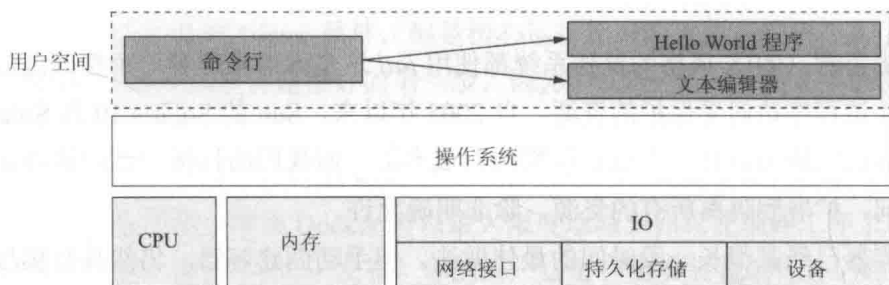
图 1-1 运行由命令行启动的两个应用所需的程序栈
