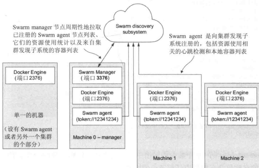
图 12-4 Swarm manager 和代理通过集群发现子系统交互
