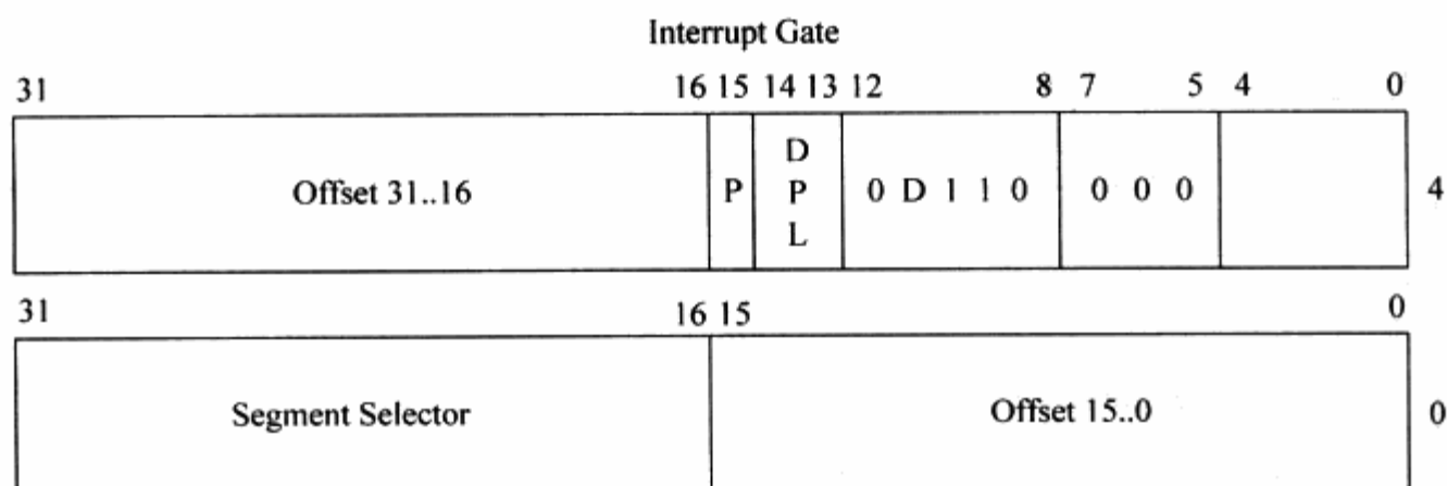
图 2-12 中断门
