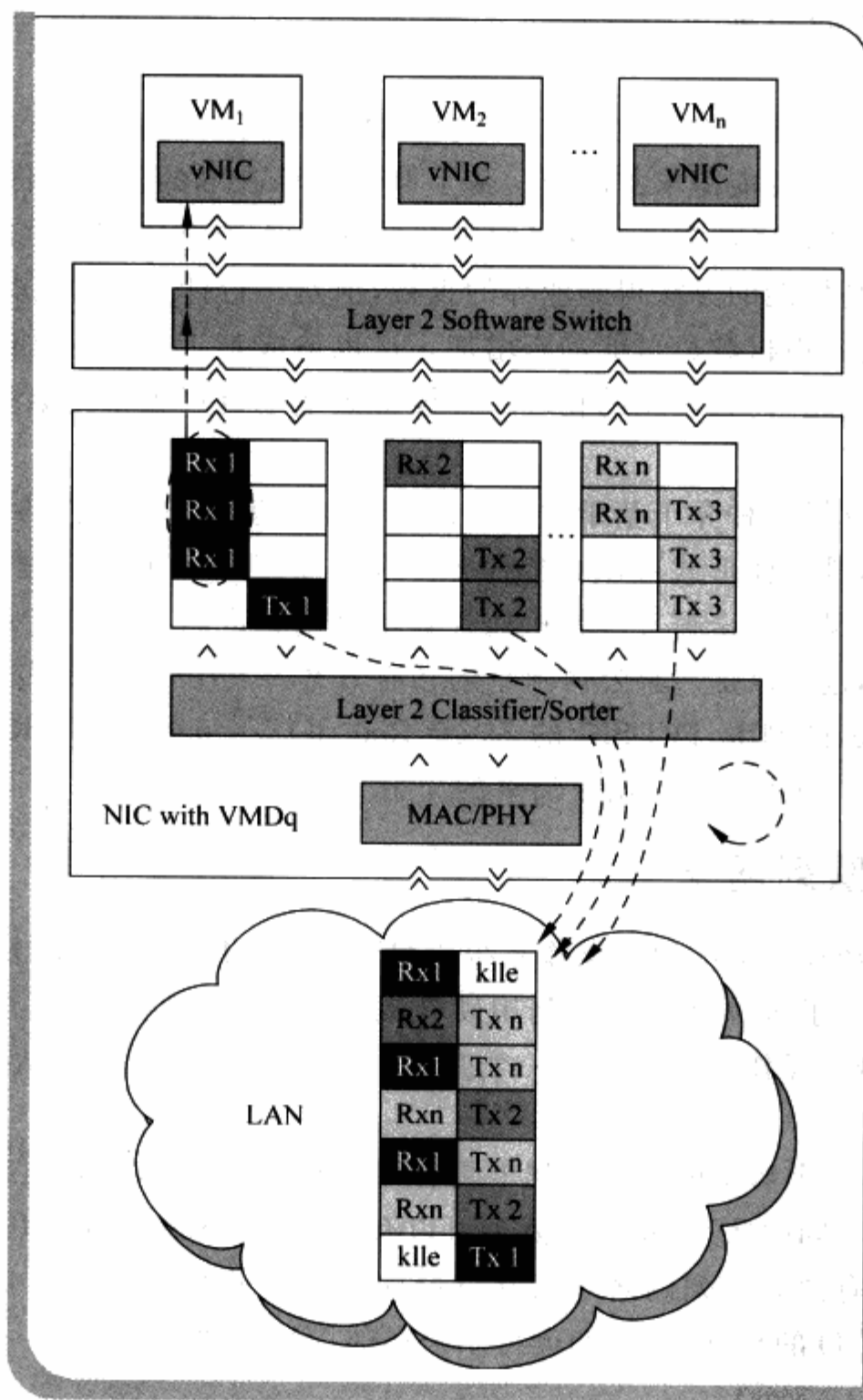
图 9-5 多列队网卡
