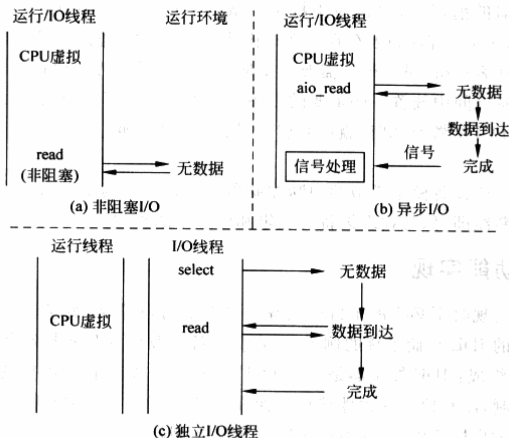
图 4-20 设备模型的 I/O 模型
