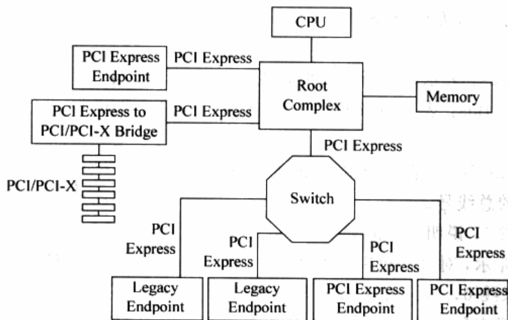
图 2-18 PCI Express 拓扑结构图
